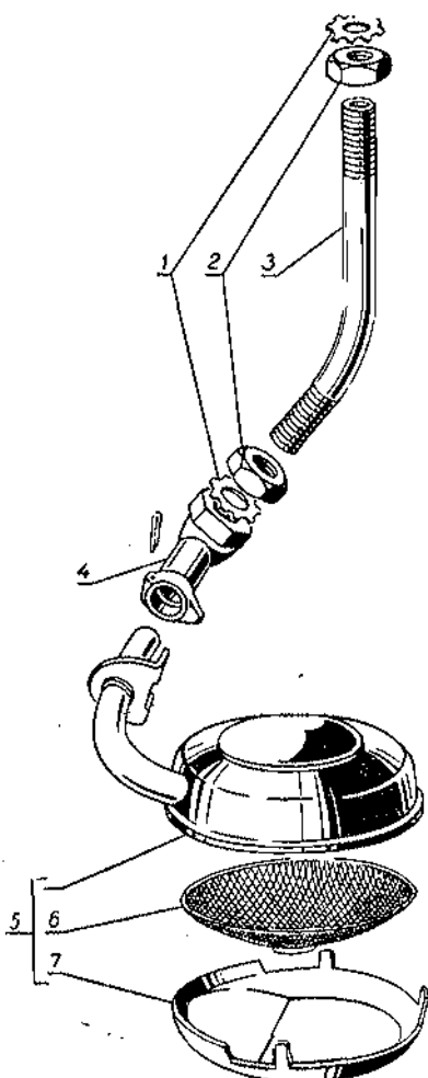
Фиг. 15. Маслоприемник.
