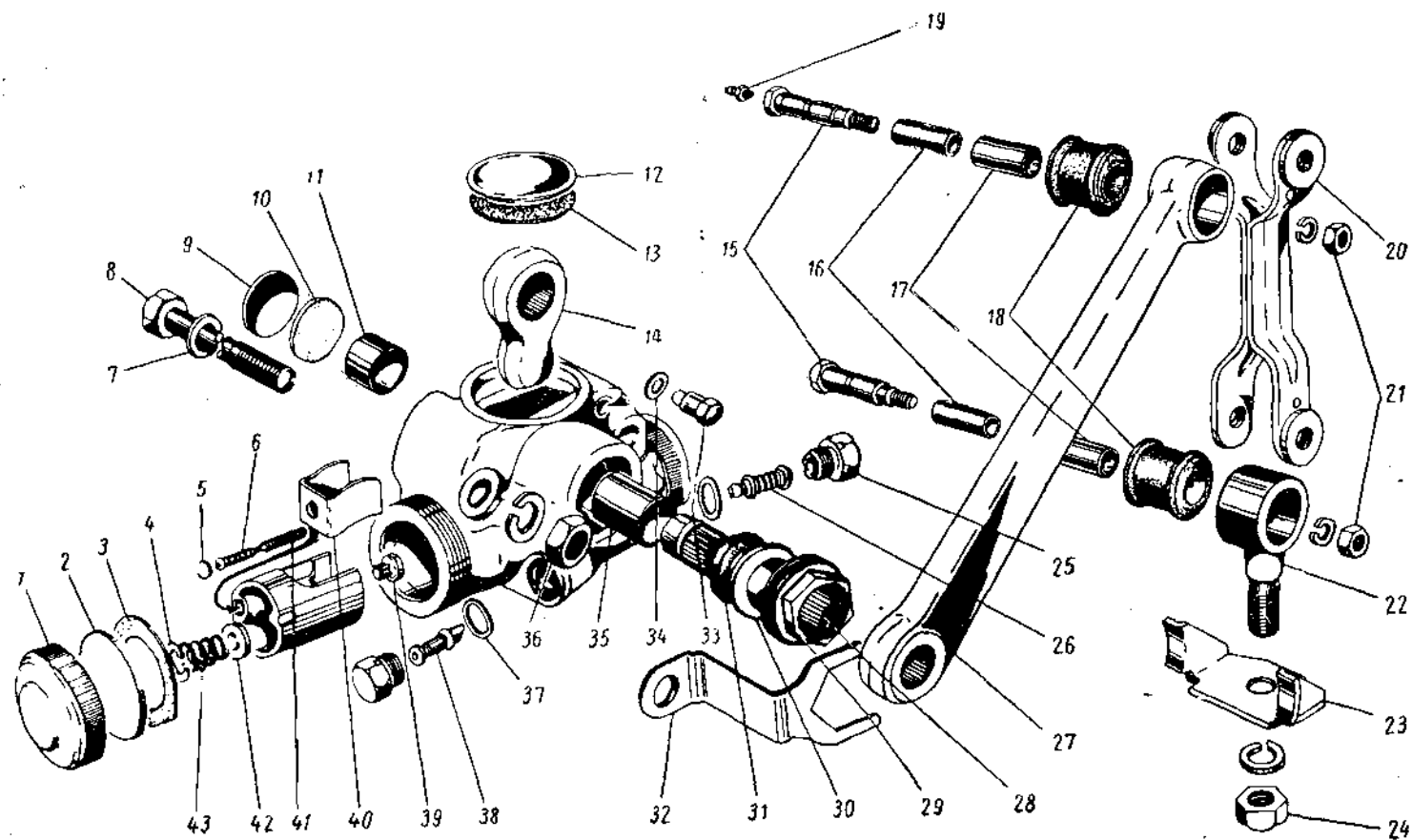
Фиг. 61. Амортизатор задней подвески.
