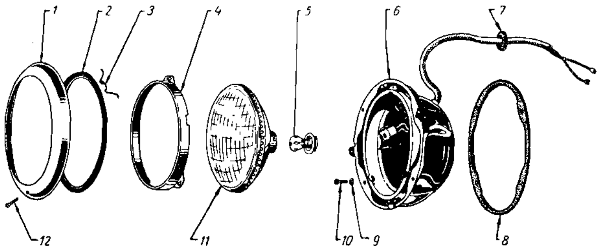
Фиг. 79. Фара
