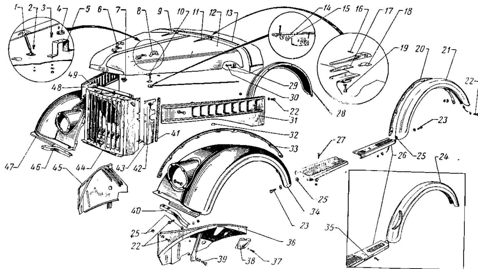
Фиг. 107. Детали оперения автомобилей ГАЗ-69 и ГАЗ-69А.
