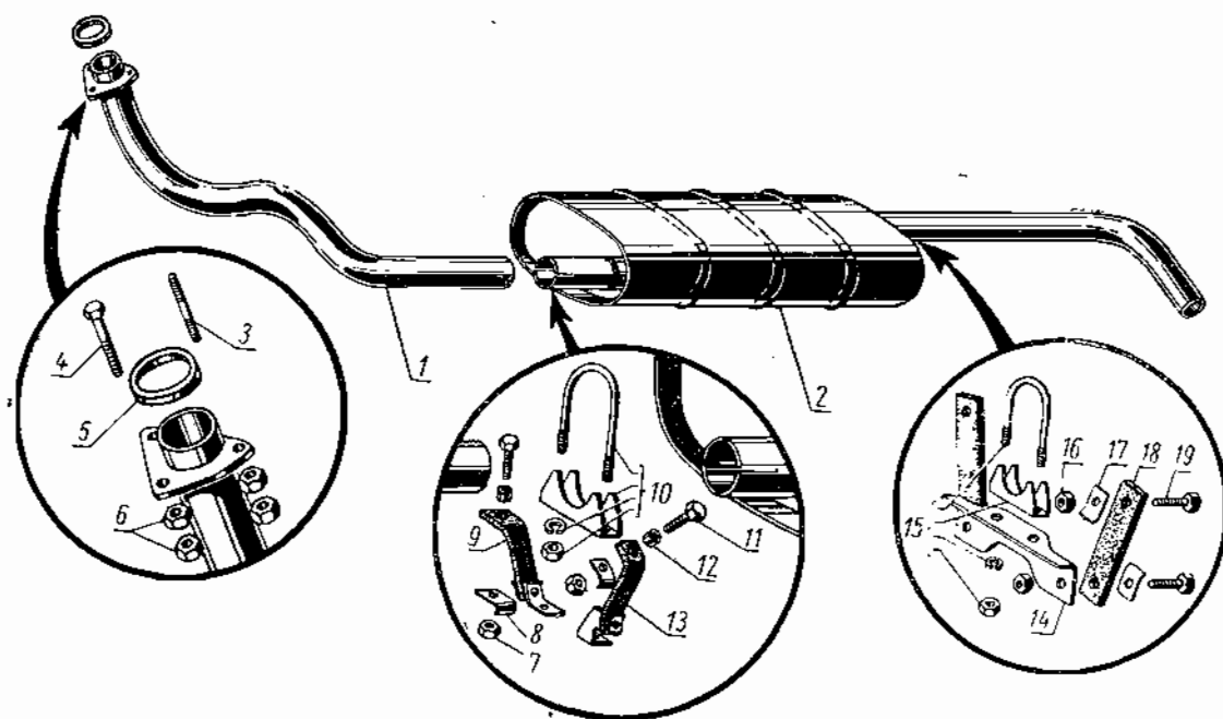
Фиг. 34. Глушитель автомобилей ГАЗ-69 и ГАЗ-69А.
