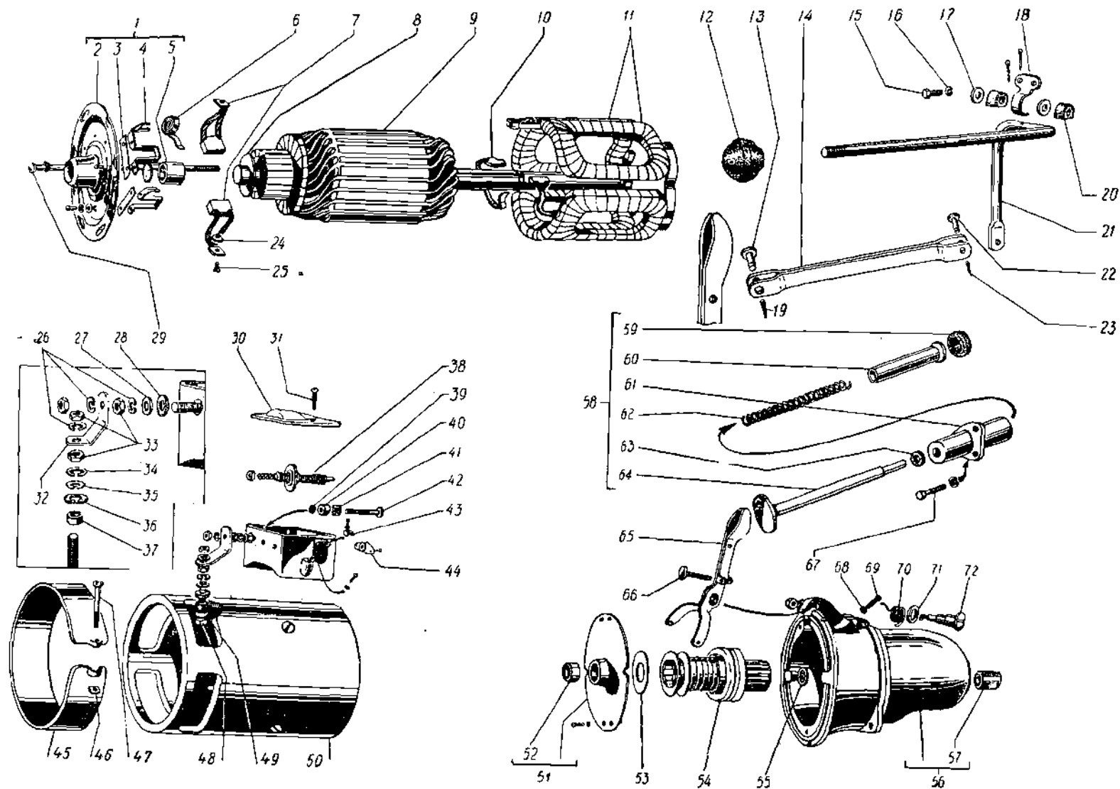
Фиг. 78. Стартёр.
