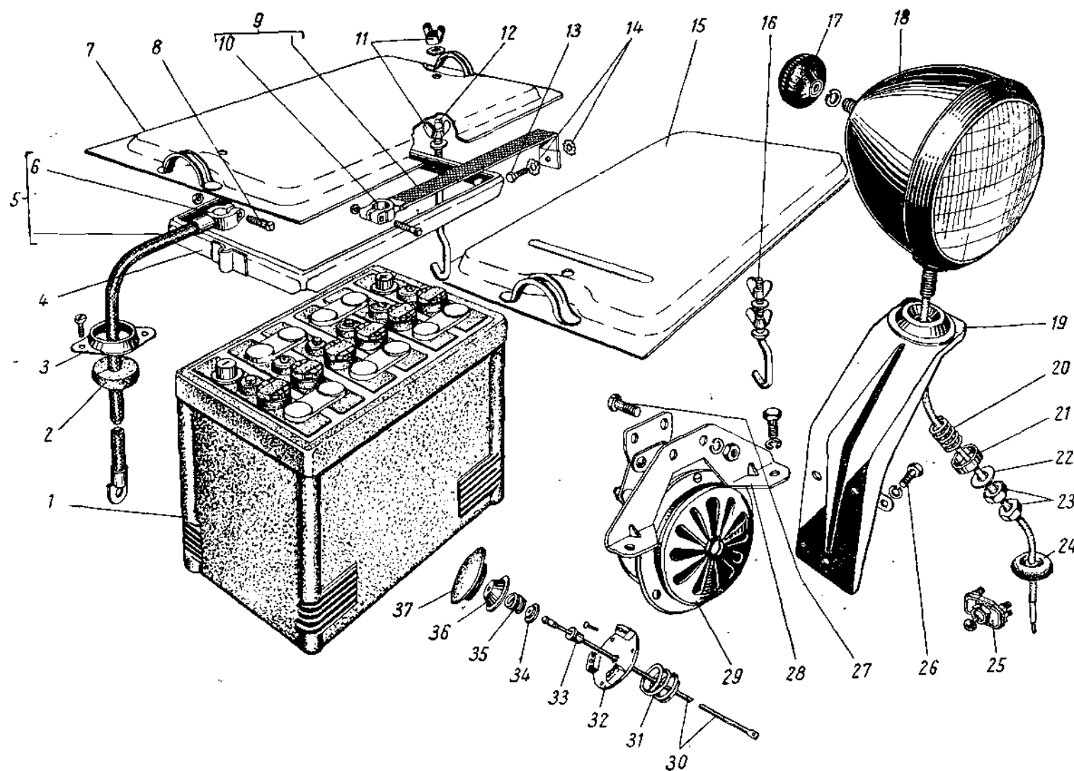
Фиг. 74. Аккумуляторная батарея, поворотная фара, сигнал и кнопка сигнала автомобилей ГАЗ-69 и ГАЗ-69А.
