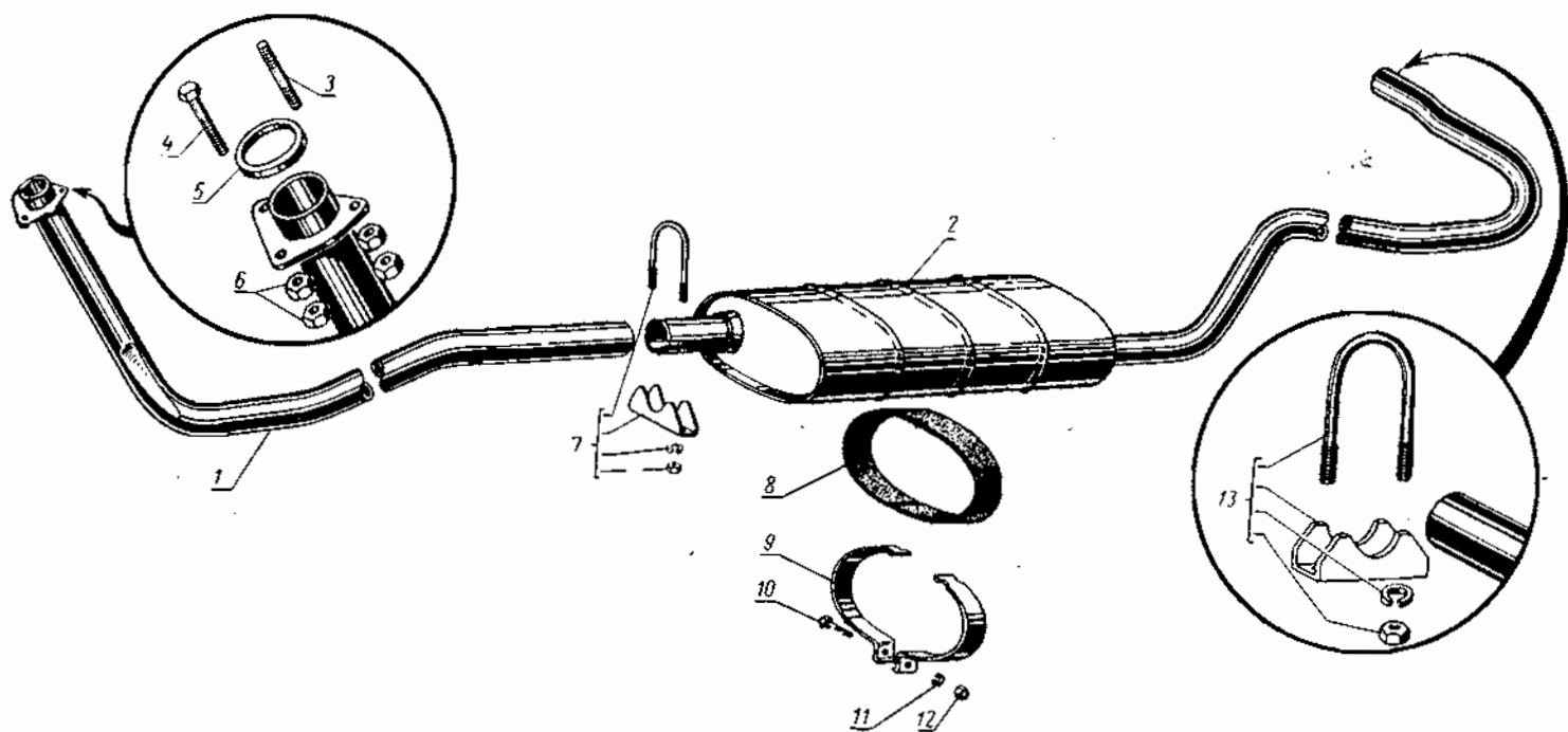
Фиг. 35. Глушитель автомобилей УАЗ-450 и УАЗ-450А.
