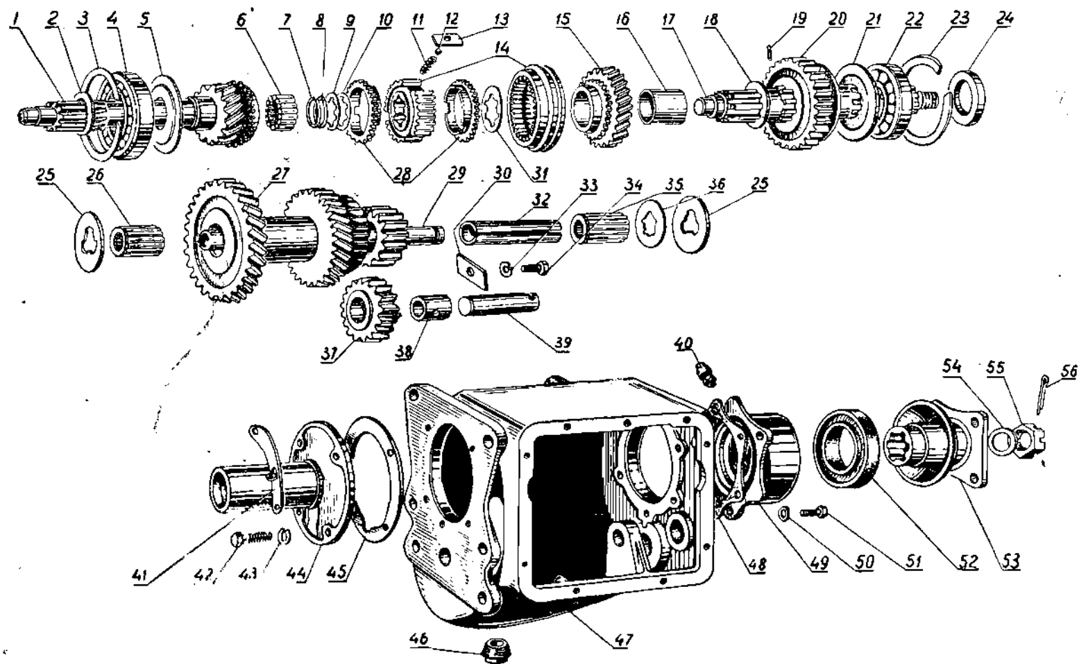
Фиг. 43. Коробка передач.
