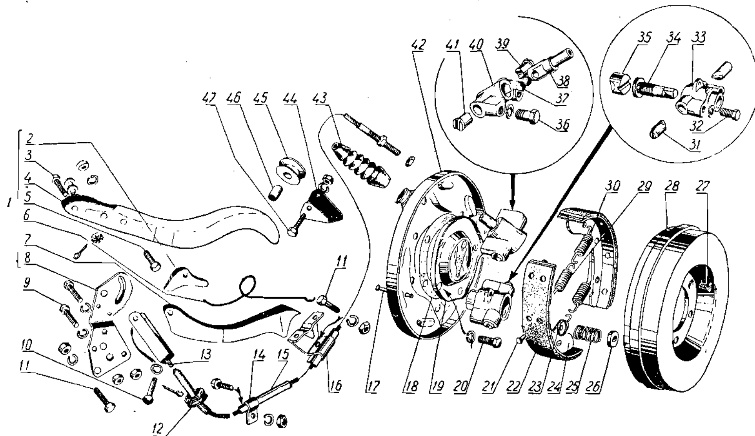
Фиг. 70. Ручной (центральный) тормоз и управление тормозом автомобилей УАЗ-450, УАЗ-450А и УАЗ-450Д
