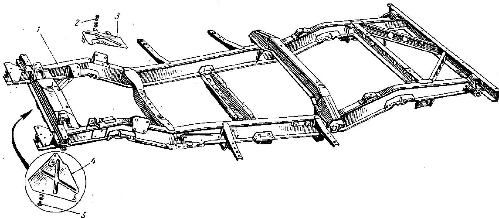
Фиг. 53. Рама автомобилей ГАЗ-69 и ГАЗ-69А.
