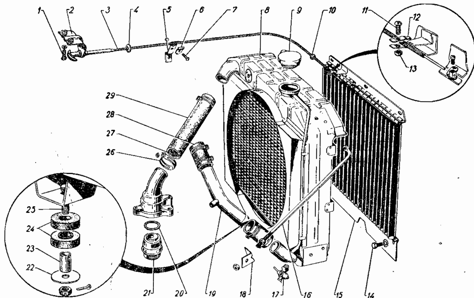
Фиг. 37. Радиатор автомобилей ГАЗ-69 и ГАЗ-69А Примечание: поз. 1-7 и 10-15 см. в подгруппе 1310.
