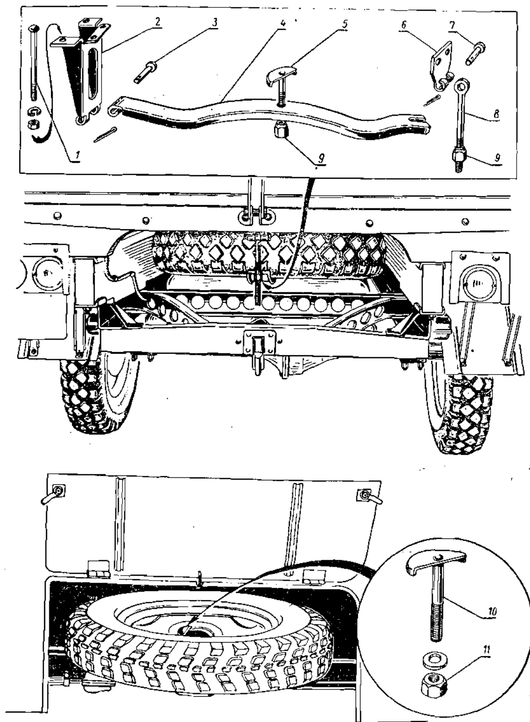
Фиг. 65. Держатель запасного колеса автомобилей УАЗ-450, УАЗ-450А и УАЗ-450Д.
