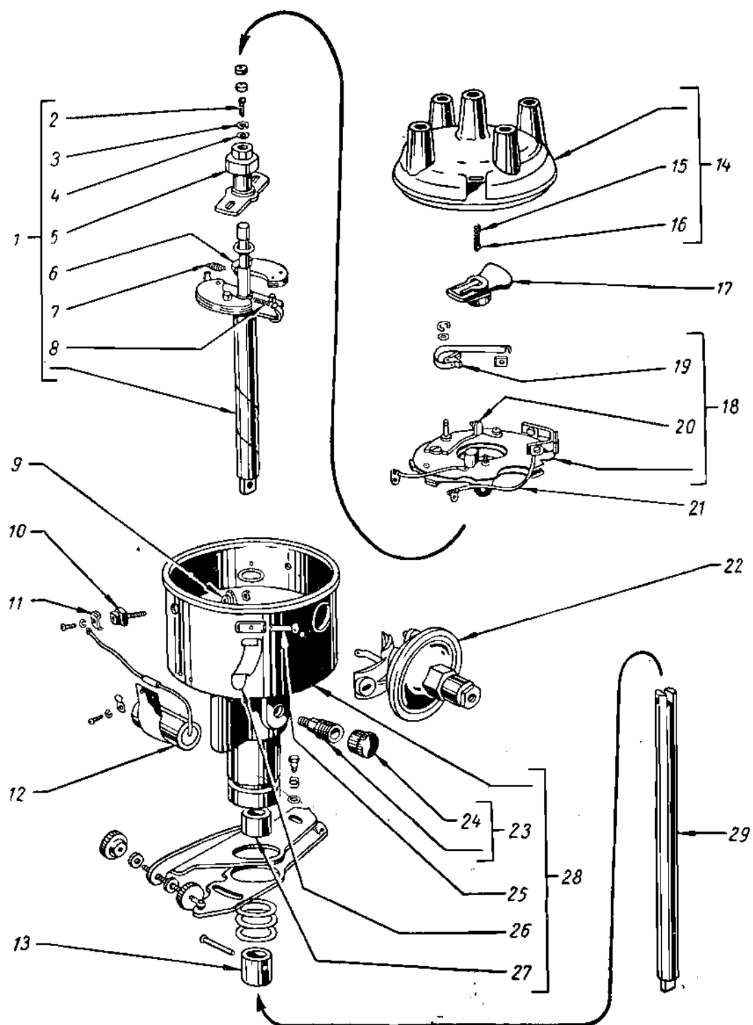
Фиг. 77. Распределитель.
