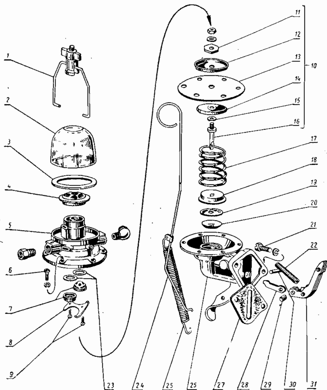
Фиг. 28. Бензиновый насос.
