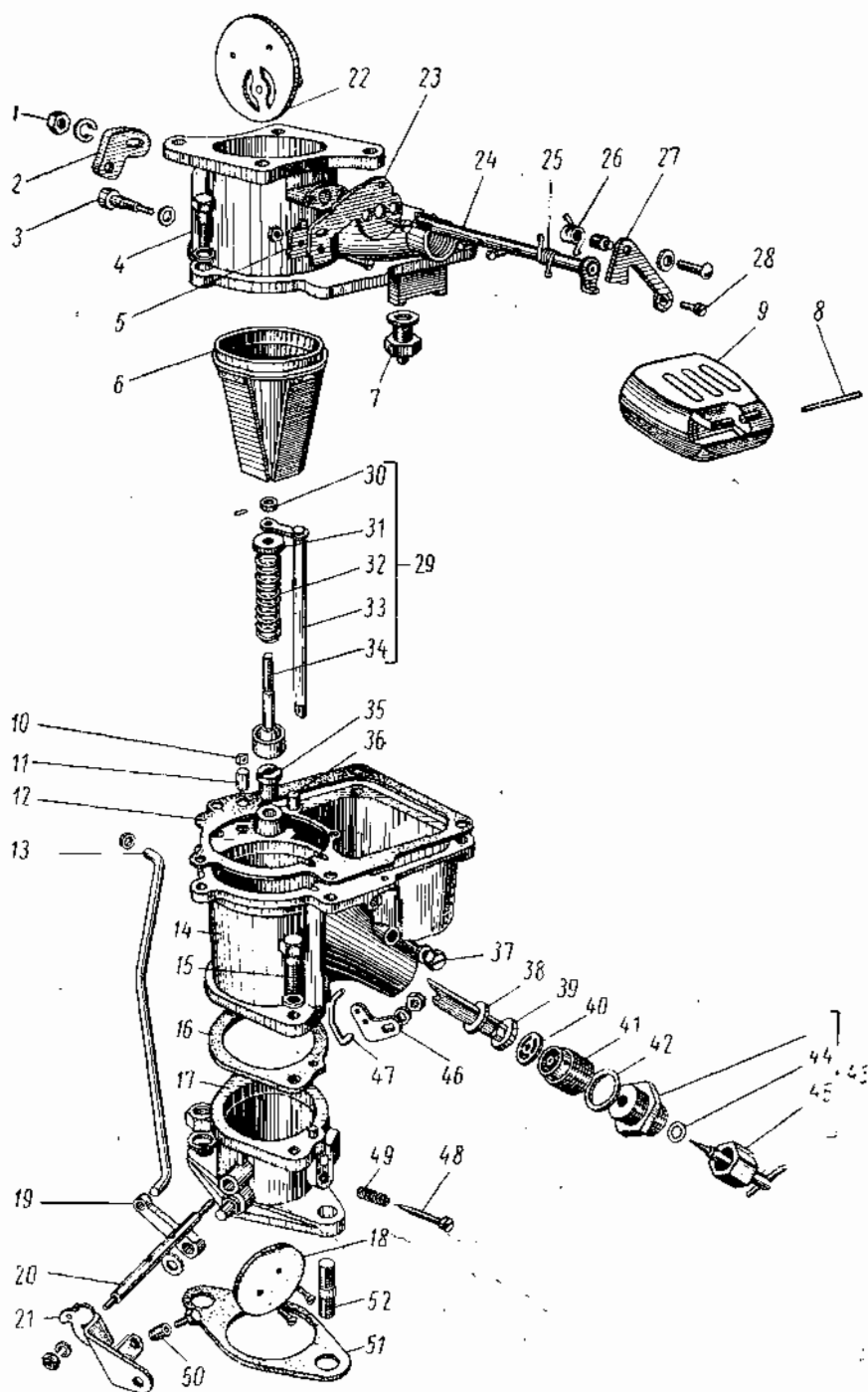
Фиг. 29. Карбюратор.
