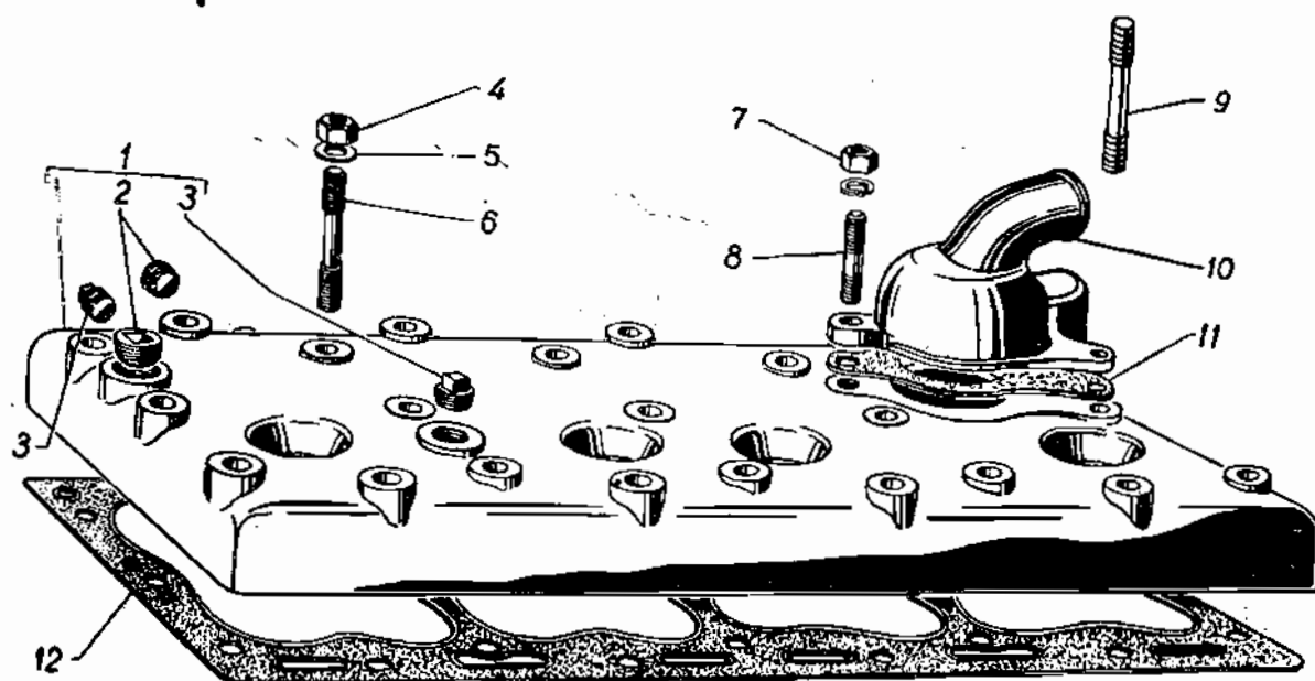
Фиг. 8. Головка блока цилиндров.
