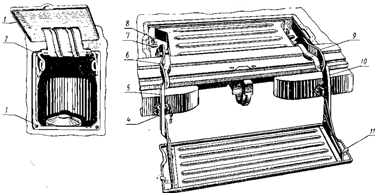
Фиг. 97. Лючки горловины бензобака автомобилей УАЗ-450 и УАЗ-450А и задняя подножка автомобиля УАЗ-450А.
