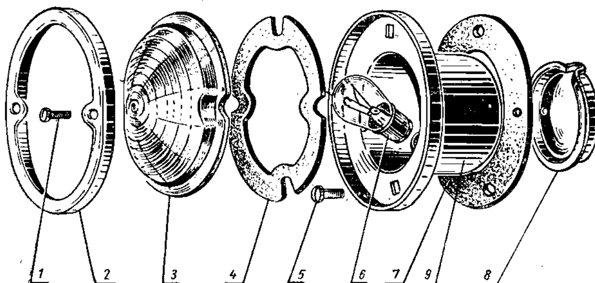
Фиг. 81. Подфарник автомобилей УАЗ-450, УАЗ-450А, УАЗ-450Д и задний фонарь (указатель поворота) автомобилей ГАЗ-69, ГАЗ-69А и УАЗ-450Д.
