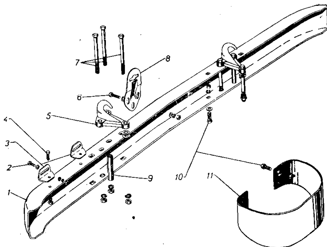
Фиг. 55. Буферы автомобилей ГАЗ-69 и ГАЗ-24.
