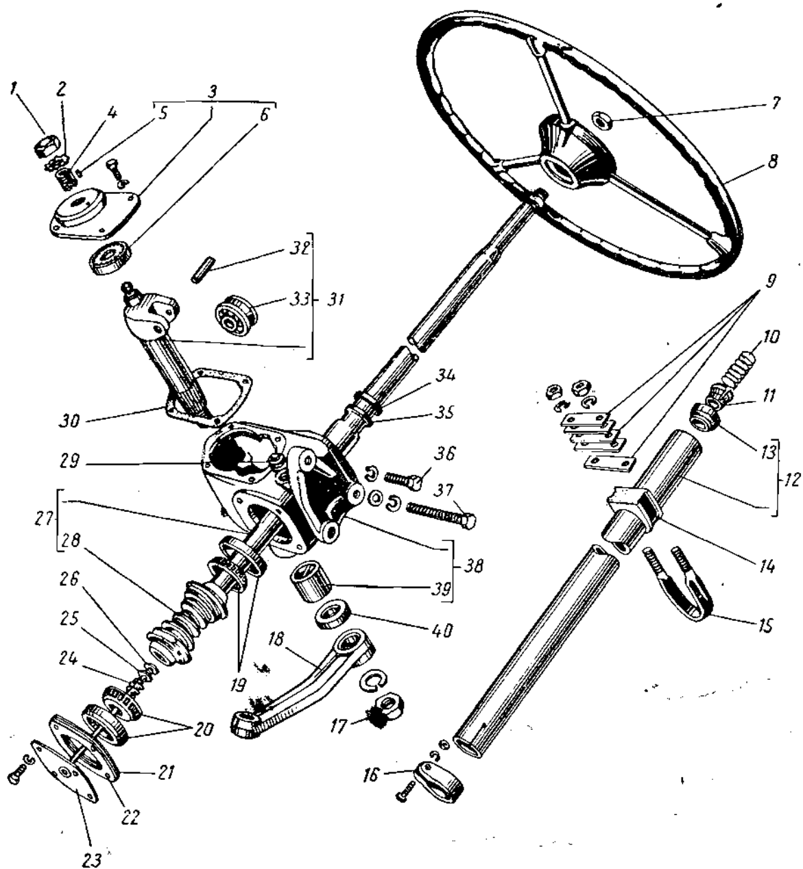
Фиг. 66. Рулевое управление автомобилей ГАЗ-69 и ГАЗ-69А.
