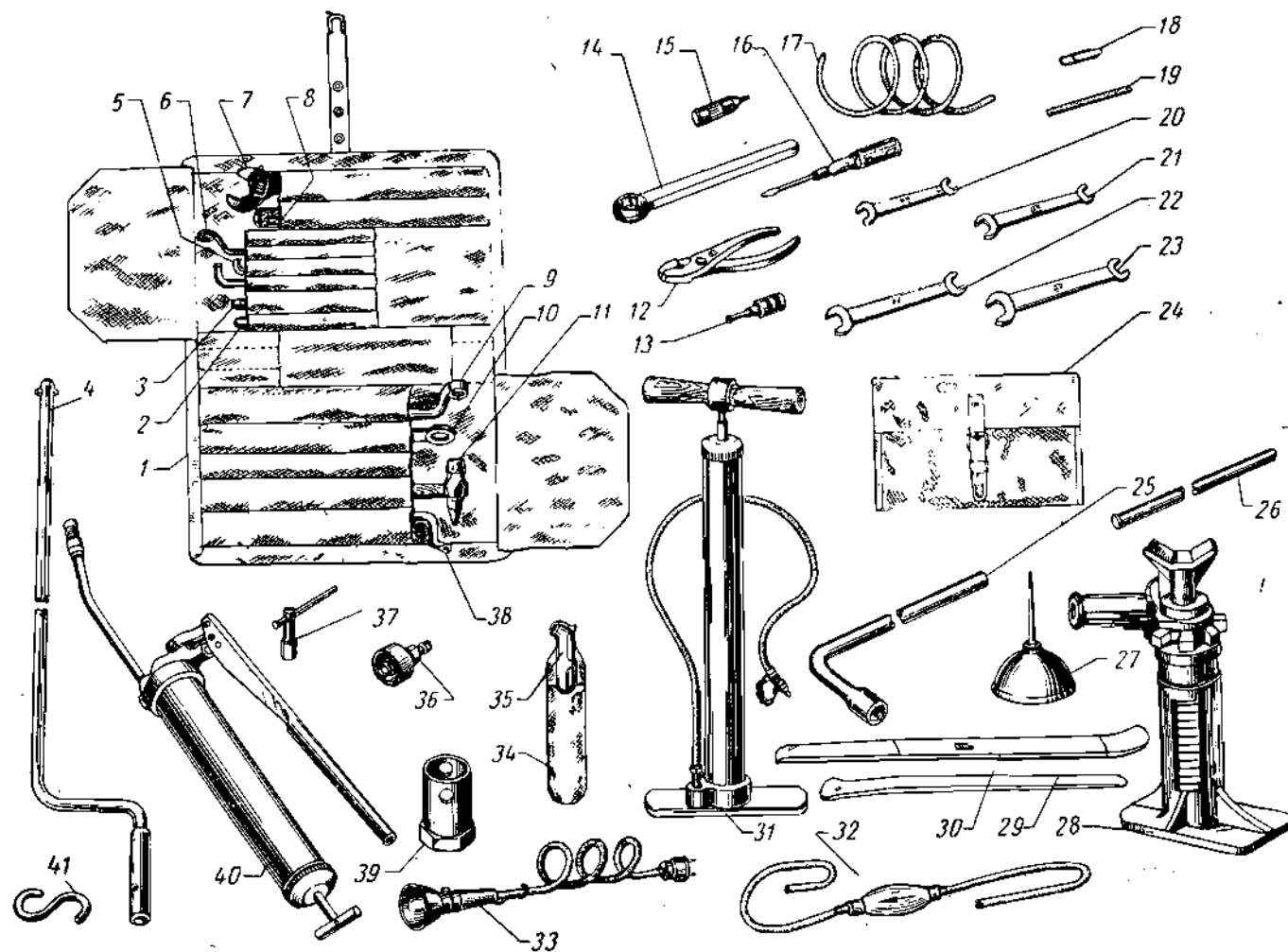
Фиг. 88. Шоферский инструмент.
