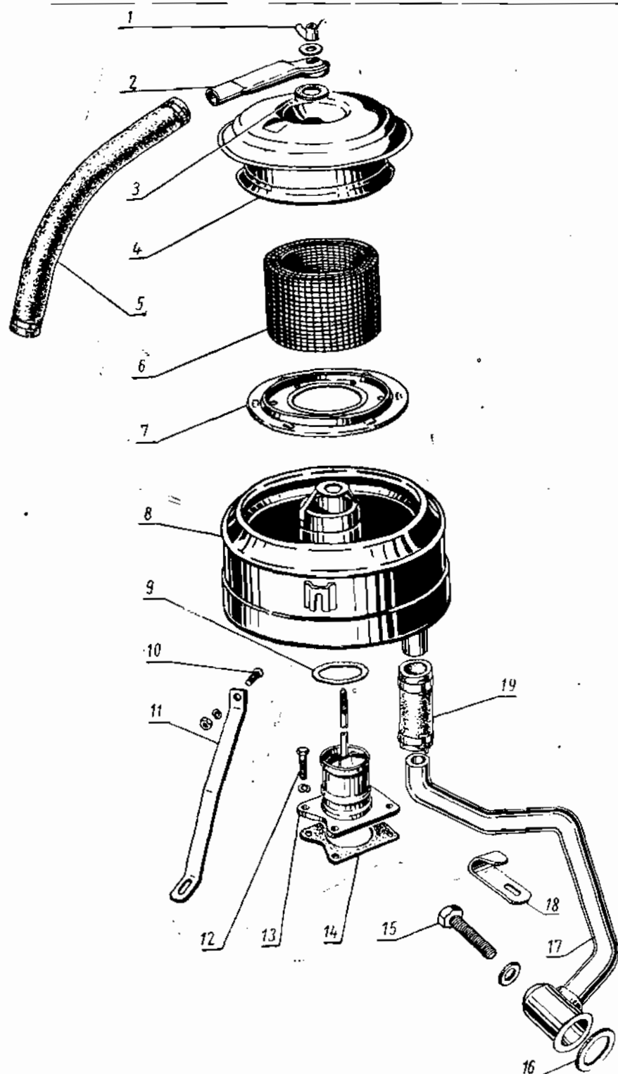
Фиг. 32. Воздушный фильтр автомобилей ГАЗ-69 и ГАЗ-69А.
