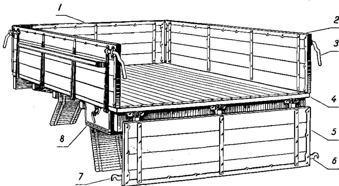
Фиг. 108. Платформа автомобиля УАЗ-450Д.
