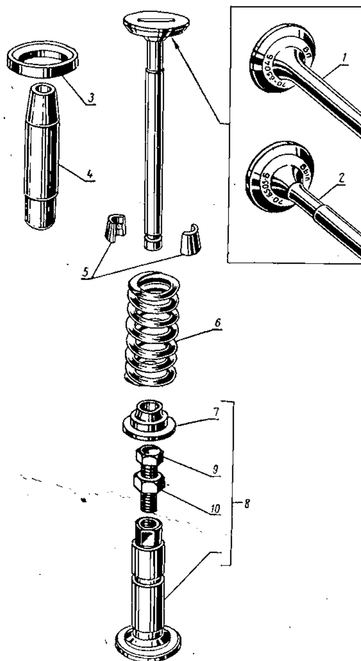
Фиг. 12. Клапаны и толкатели.
