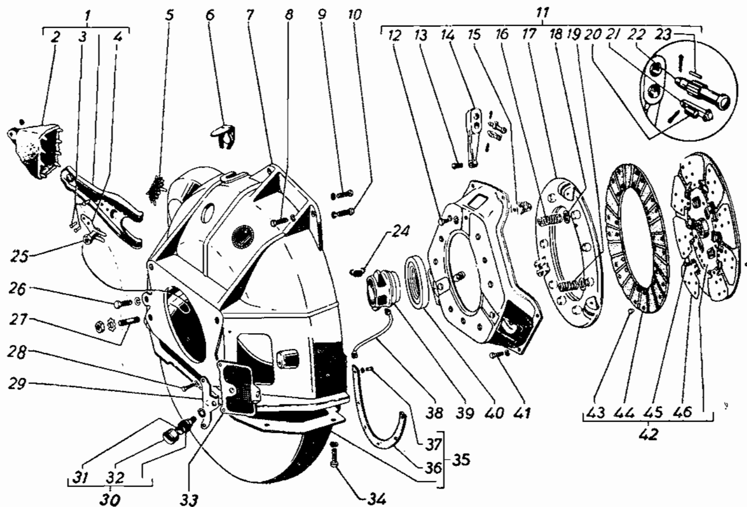
Фиг. 40. Сцепление.
