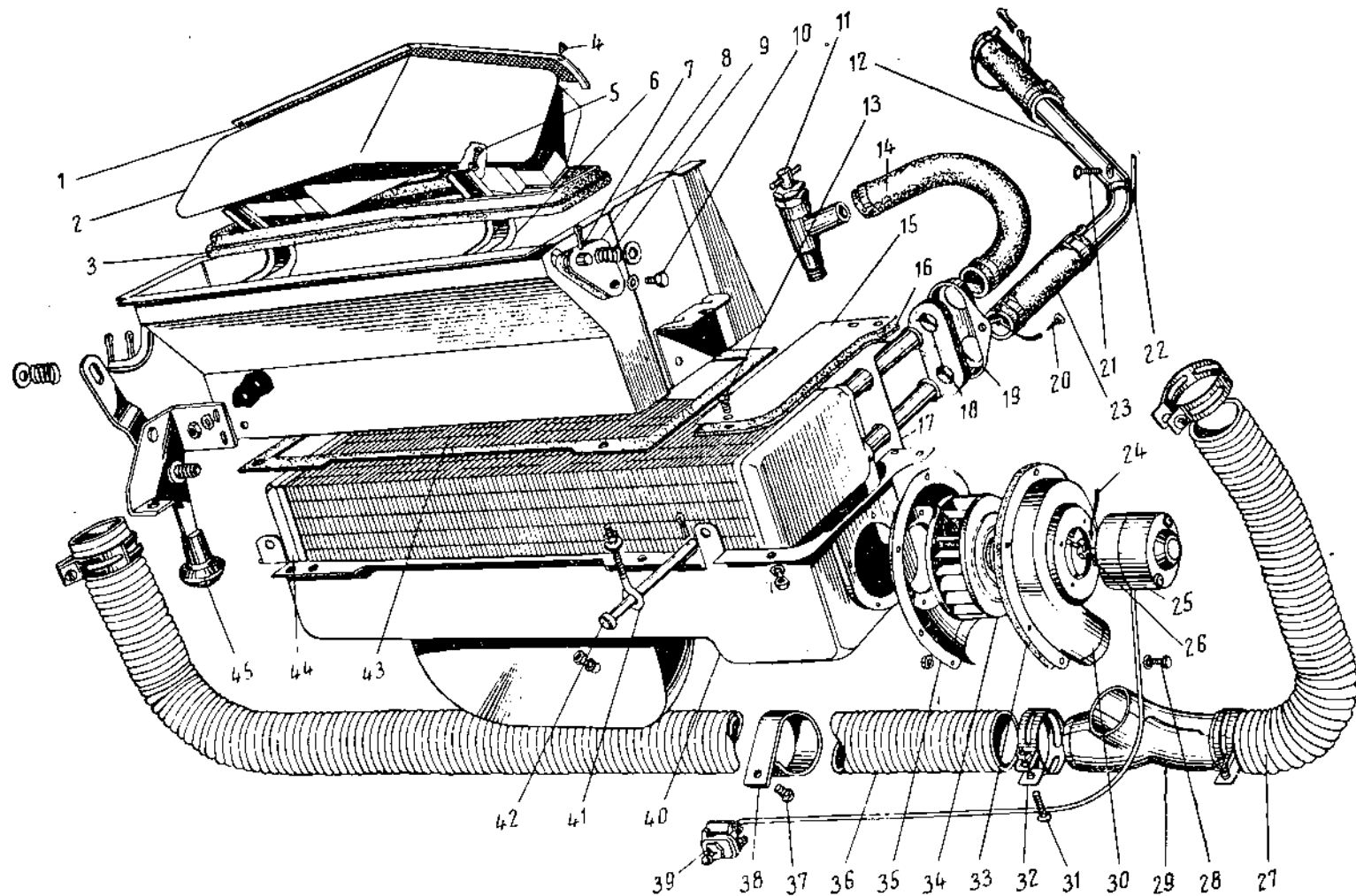
Фиг. 96. Вентиляция передка и отопление кузова автомобилей ГАЗ-69 и ГАЗ-69А.
