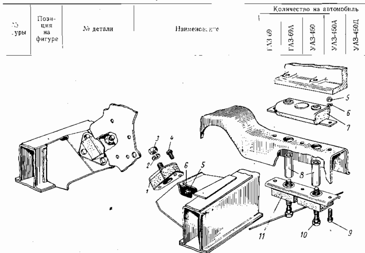
Фиг. 6. Крепление двигателя.
