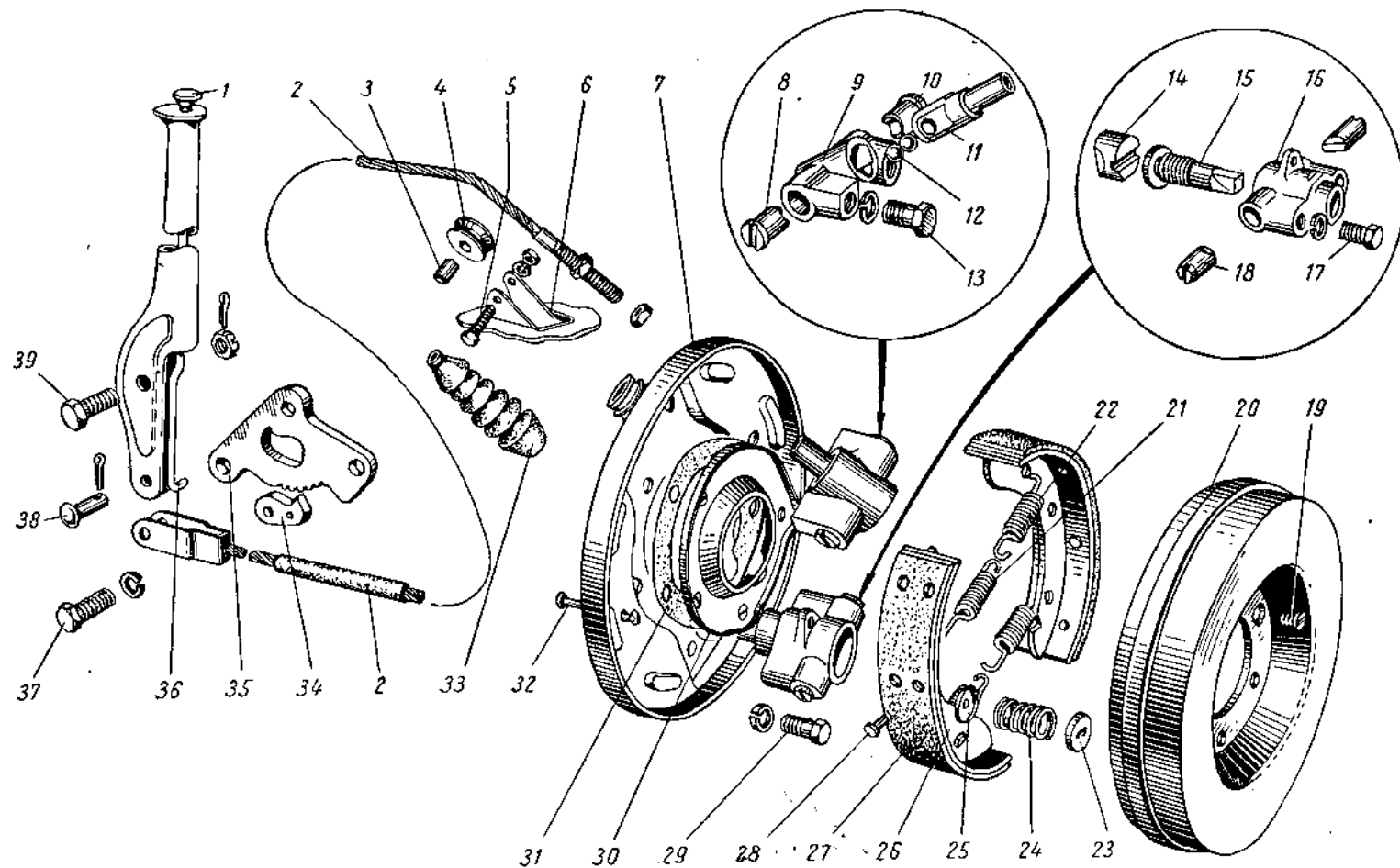
Фиг. 69. Ручной (центральный) тормоз и управление тормозом автомобилей ГАЗ-69 и ГАЗ-69А
