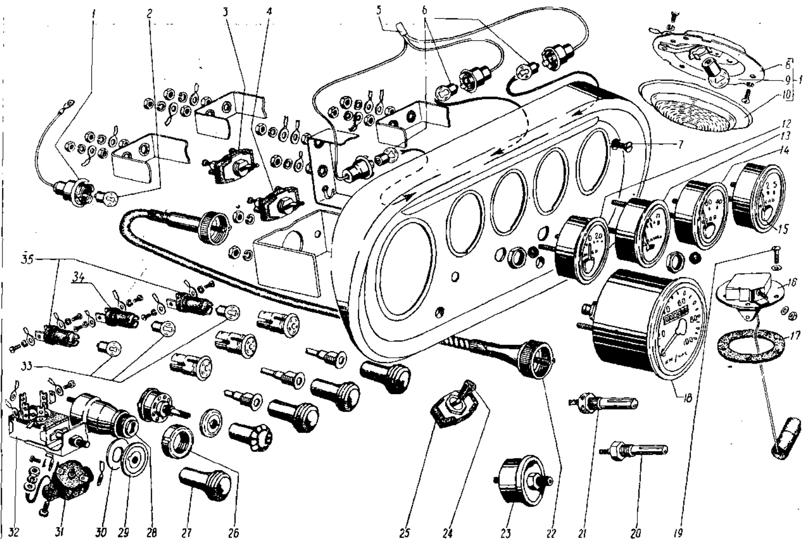
Фиг. 87. Щиток приборов и приборы автомобилей УАЗ-450, УАЗ-450А и УАЗ-450Д.
