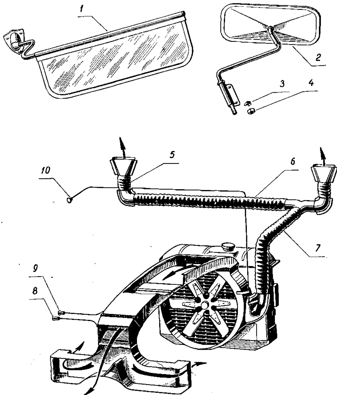
Фиг. 105. Отопление и обдув ветрового окна, зеркало заднего вида и противосолнечный козырек автомобилей УАЗ-450, УАЗ-450А и УАЗ-450Д.
