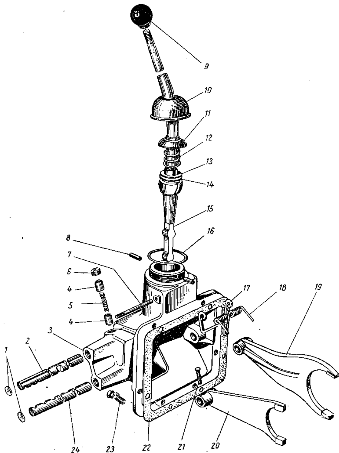
Фиг. 44. Механизм переключения передач автомобилей ГАЗ-69 и ГАЗ-69А.
