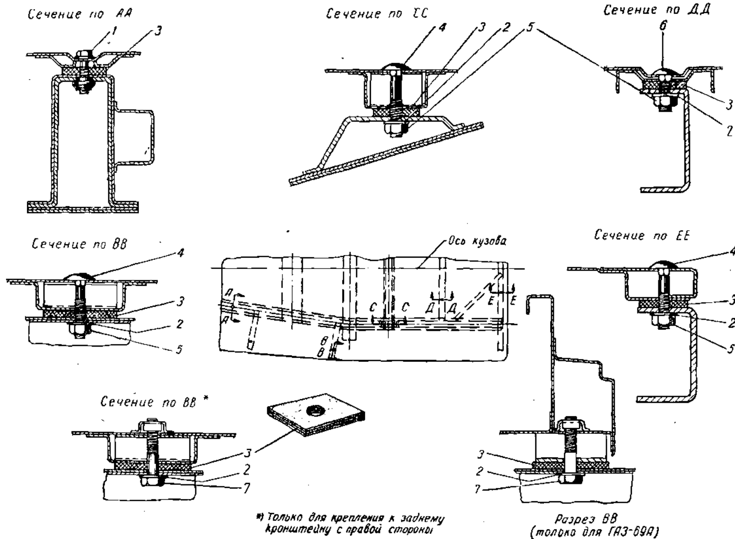
Фиг. 89. Крепление кузова автомобилей ГАЗ-69 и ГАЗ-69А.
