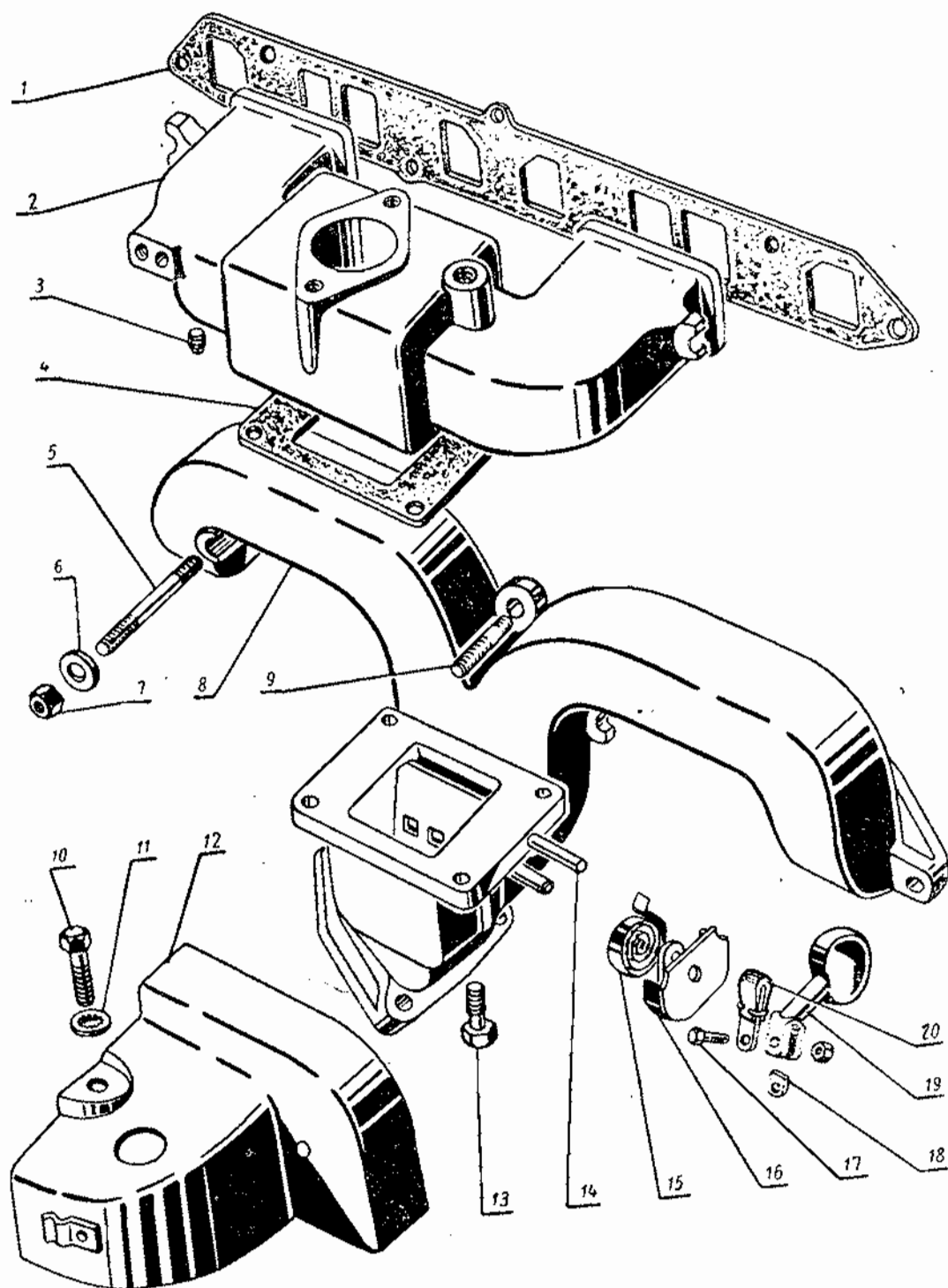
Фиг. 13. Газопровод.
