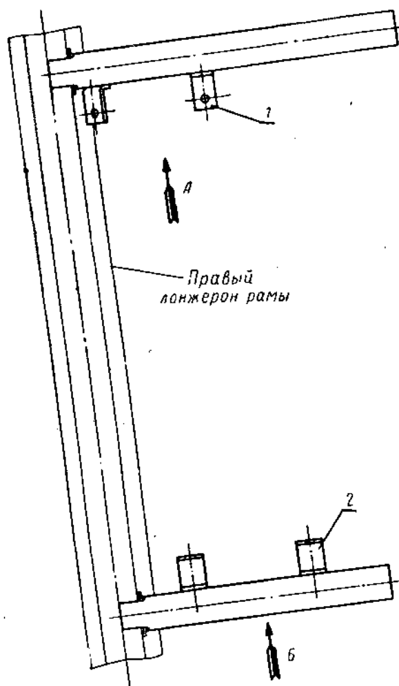
Фиг. 109. Приварка дополнительных деталей для крепления глушителя на автомобили ГАЗ-69 и ГАЗ-69А (выпуска до второй половины 1957 г.)
