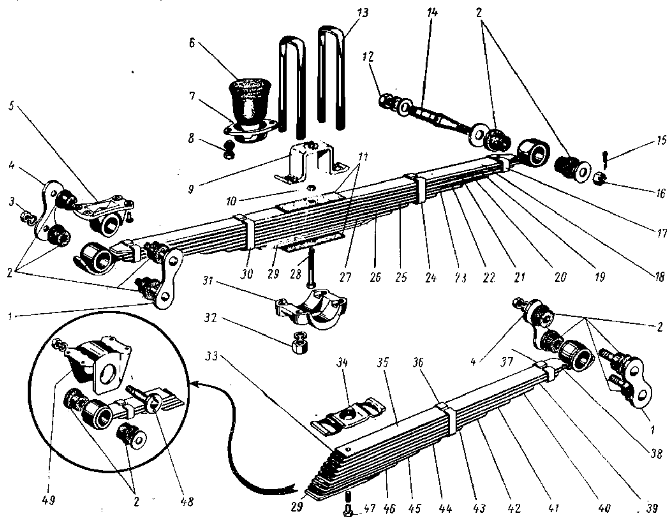
Фиг. 58. Передние и задние рессоры автомобилей ГАЗ-69 и ГАЗ-69А.
