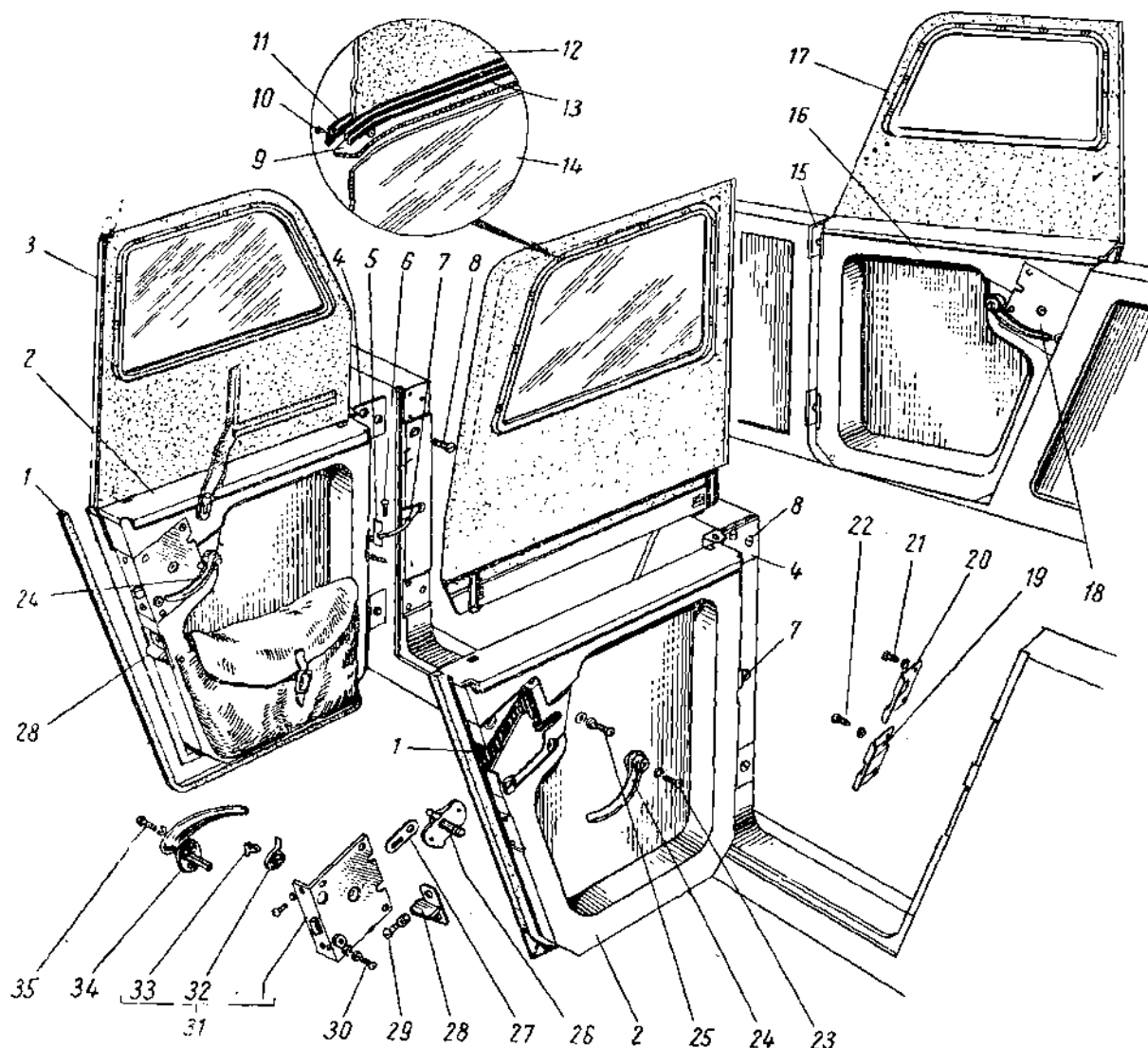
Фиг. 101. Двери кузова автомобиля ГАЗ-69А.
