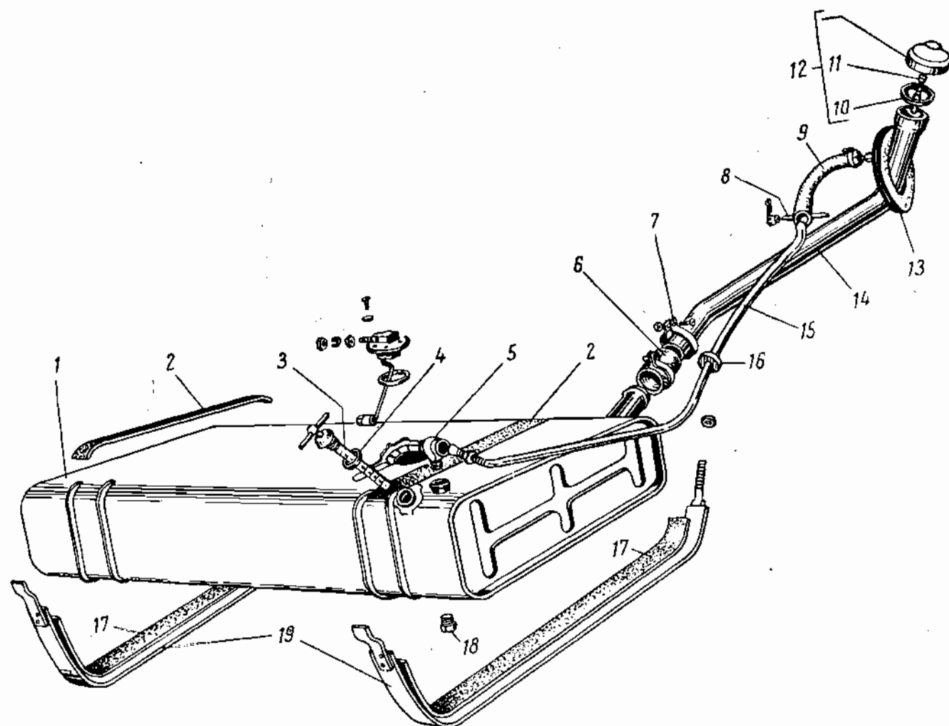
Фиг. 22. Бензиновый бак автомобиля ГАЗ-69А.
