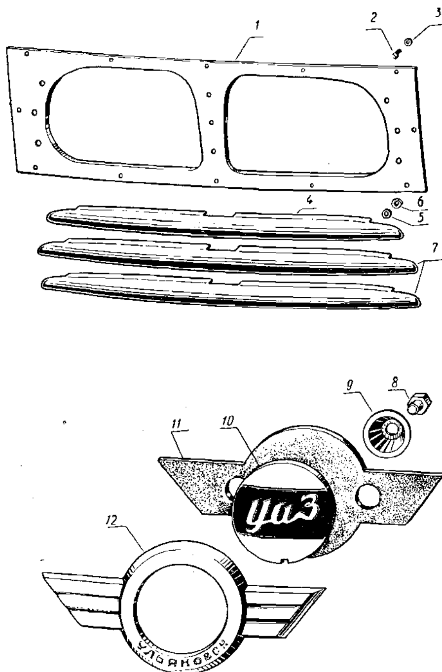
Фиг. 95. Облицовка радиатора и эмблема автомобилей УАЗ-450, УАЗ-450А и УАЗ-450Д.
