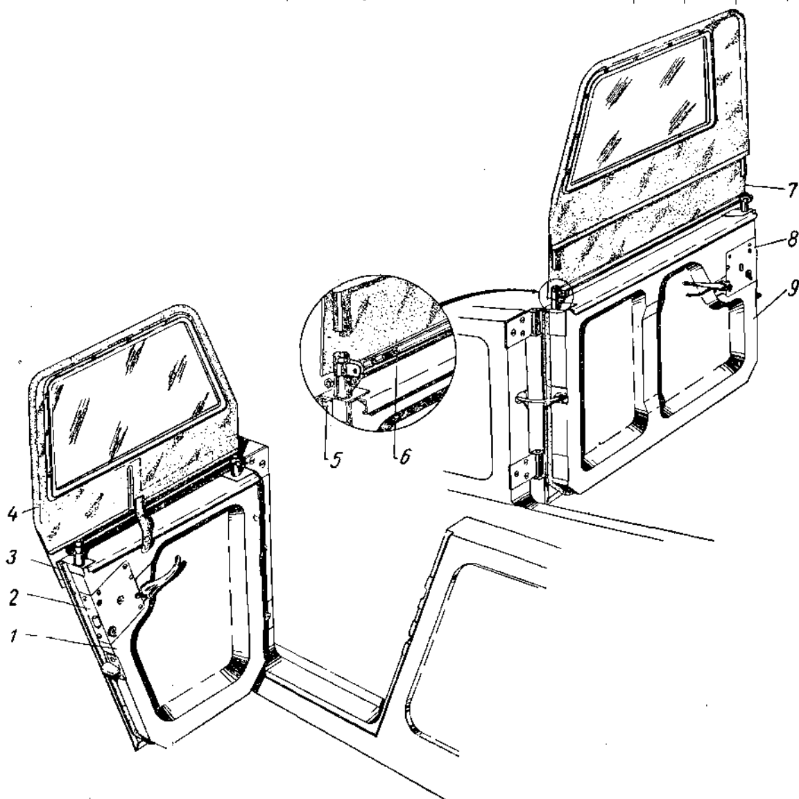
Фиг. 100. Двери кузова автомобиля ГАЗ-69.
