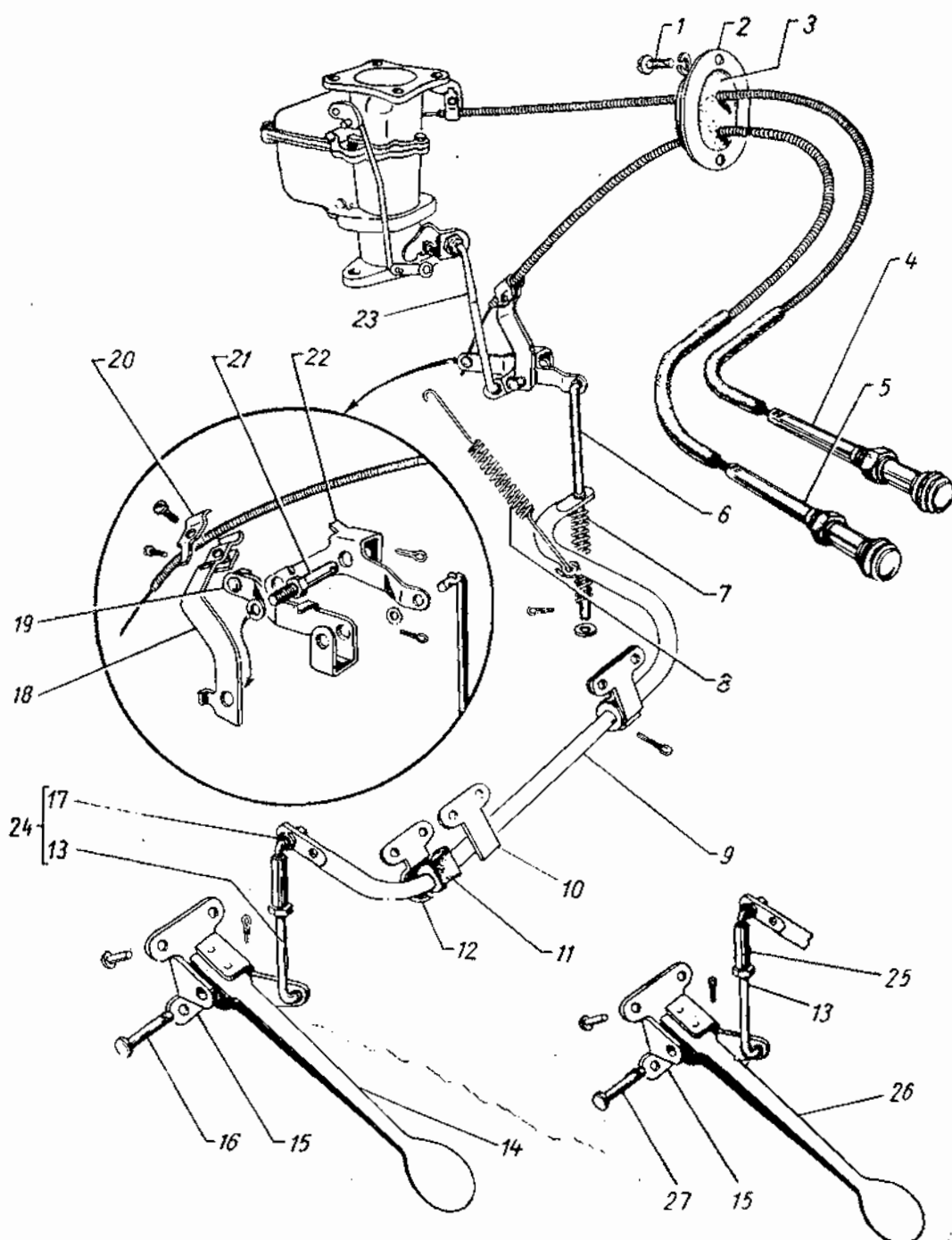
Фиг. 30. Управление карбюратором автомобилей ГАЗ-69 и ГАЗ-69А.
