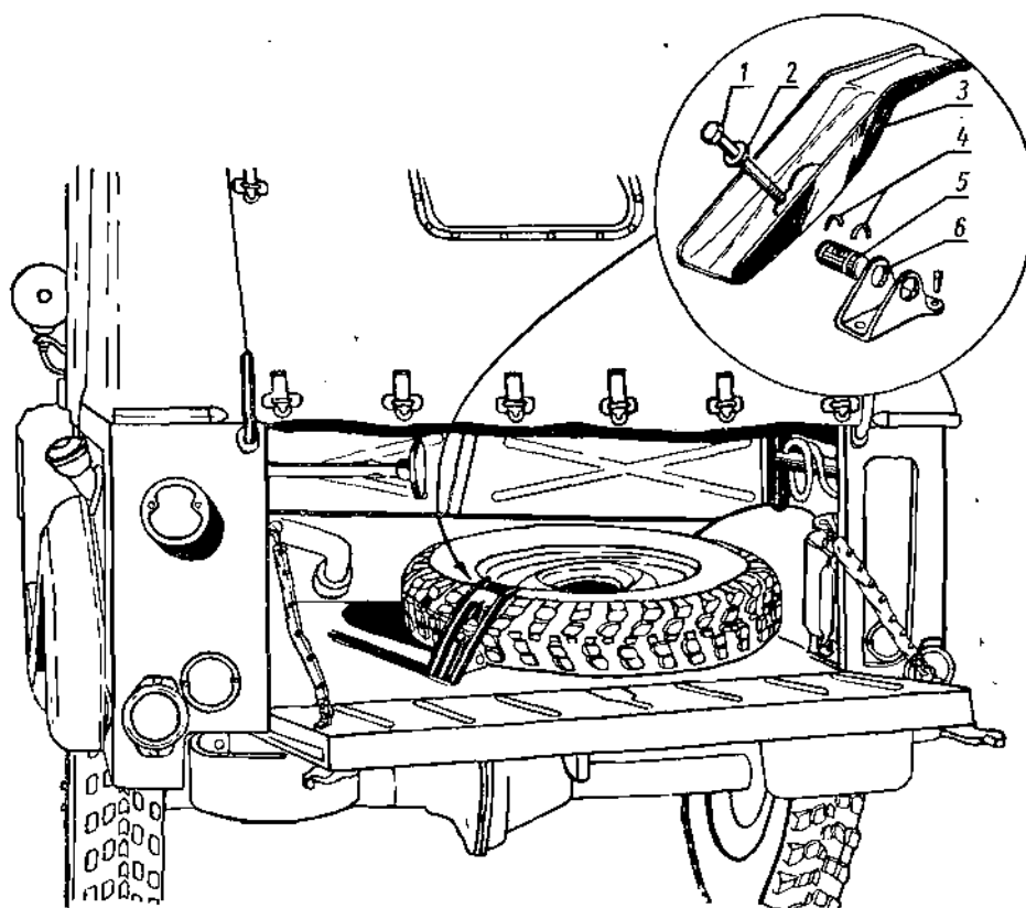
Фиг. 64. Держатель запасного колеса автомобиля ГАЗ-69А.
