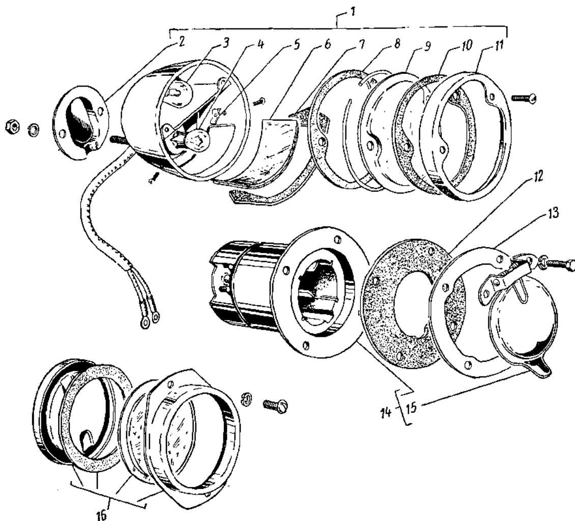
Фиг. 82. Задний фонарь автомобилей ГАЗ-69; ГАЗ-69А, УАЗ-450Д и штепсельная розетка автомобилей ГАЗ-69, ГАЗ-69А и УАЗ-450А.
