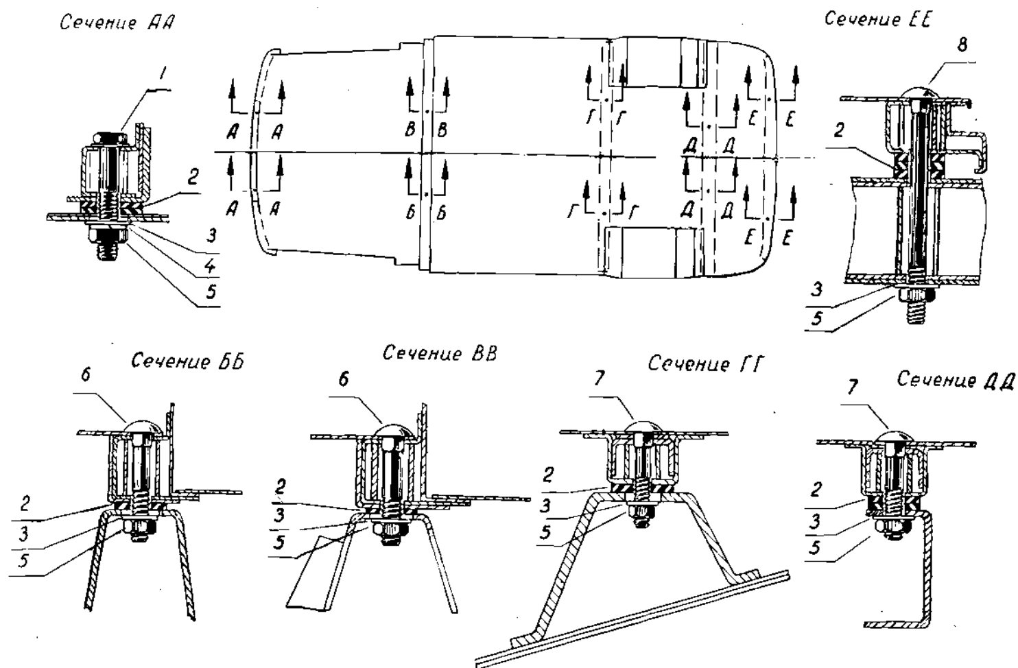
Фиг. 90. Крепление кузова автомобилей УАЗ-450, УАЗ-450А и УАЗ-450Д.
