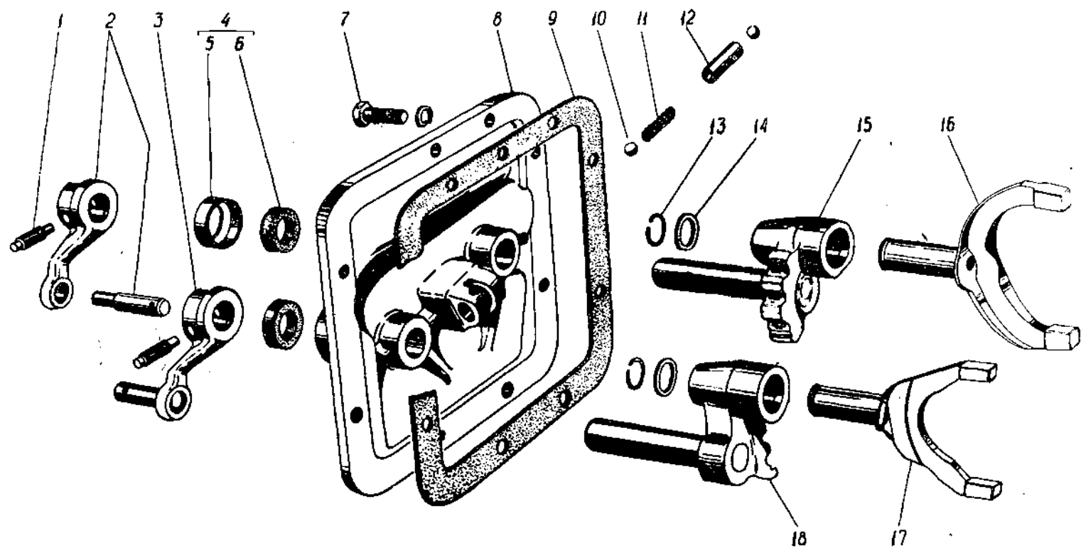
Фиг. 45. Механизм переключения передач автомобилей УАЗ-450, УАЗ-450А и УАЗ-450Д.
