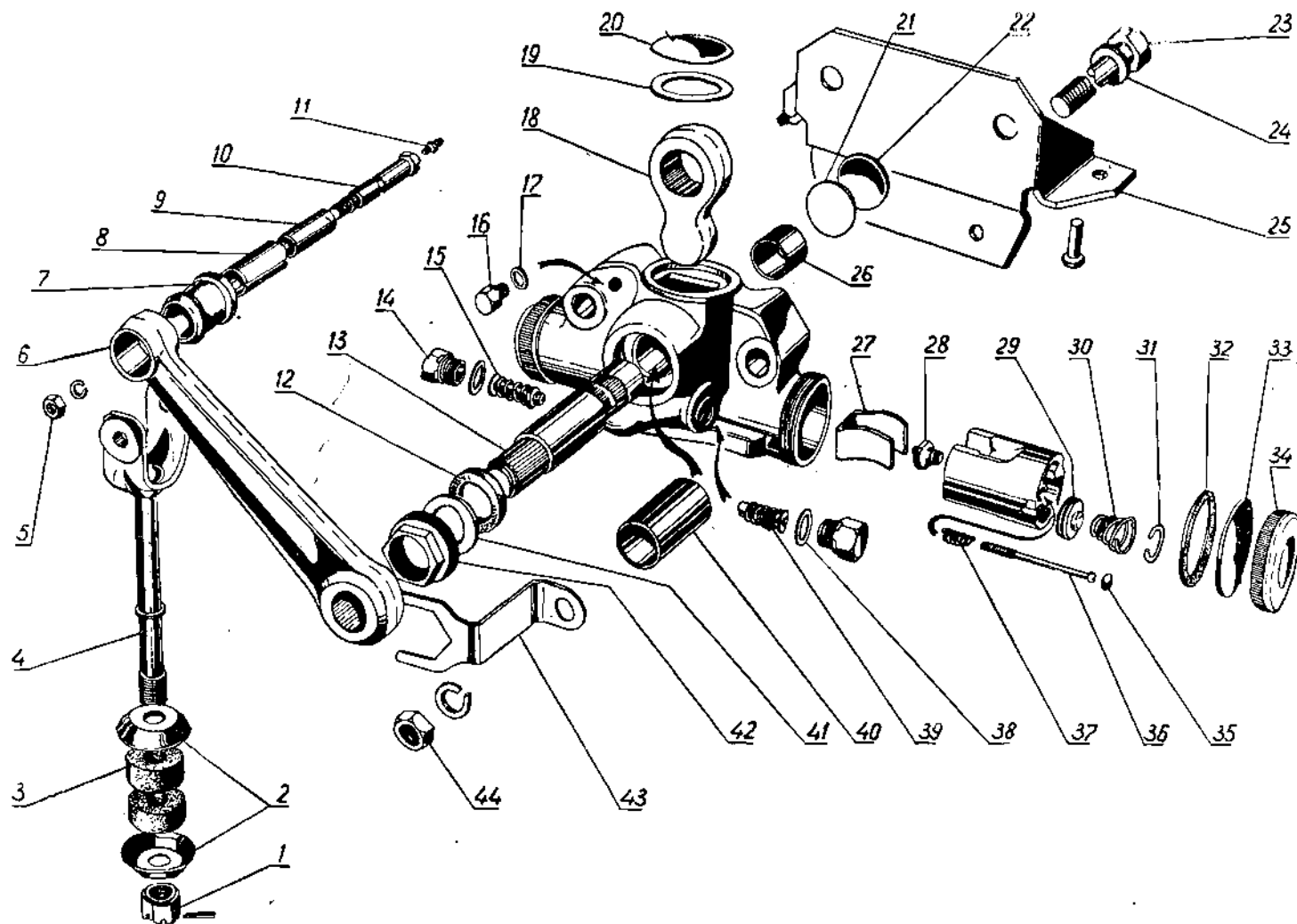
Фиг. 60. Амортизатор передней подвески.
