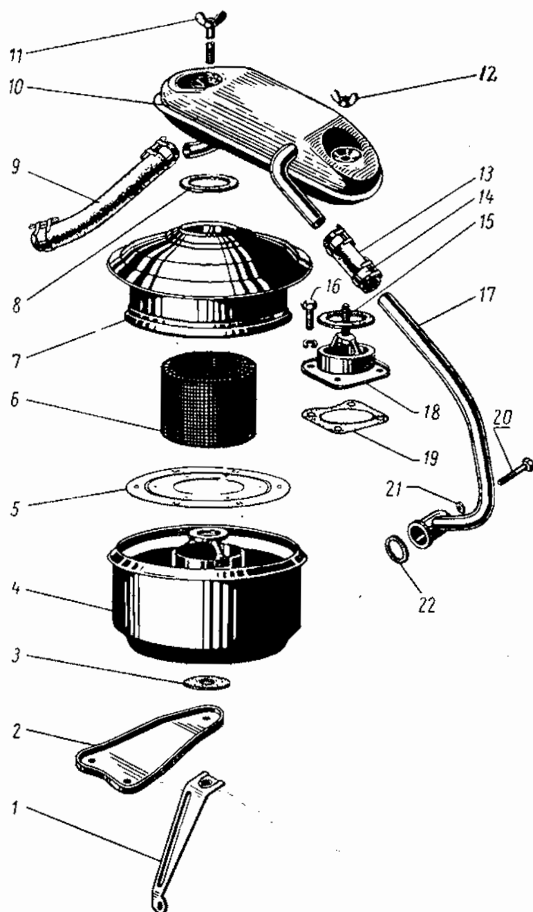
Фиг. 33. Воздушный фильтр автомобилей УАЗ-450, УАЗ-450А и УАЗ-450Д.
