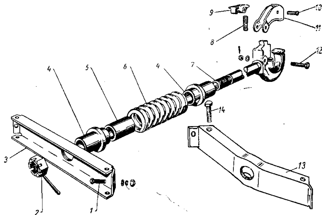
Фиг. 57. Буксирный прибор.
