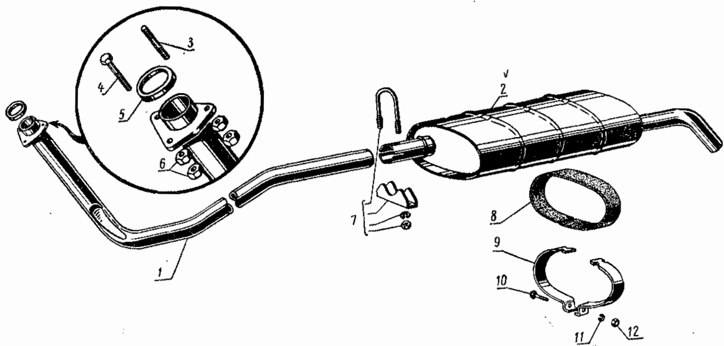
Фиг. 36. Глушитель автомобиля УАЗ-450Д.
