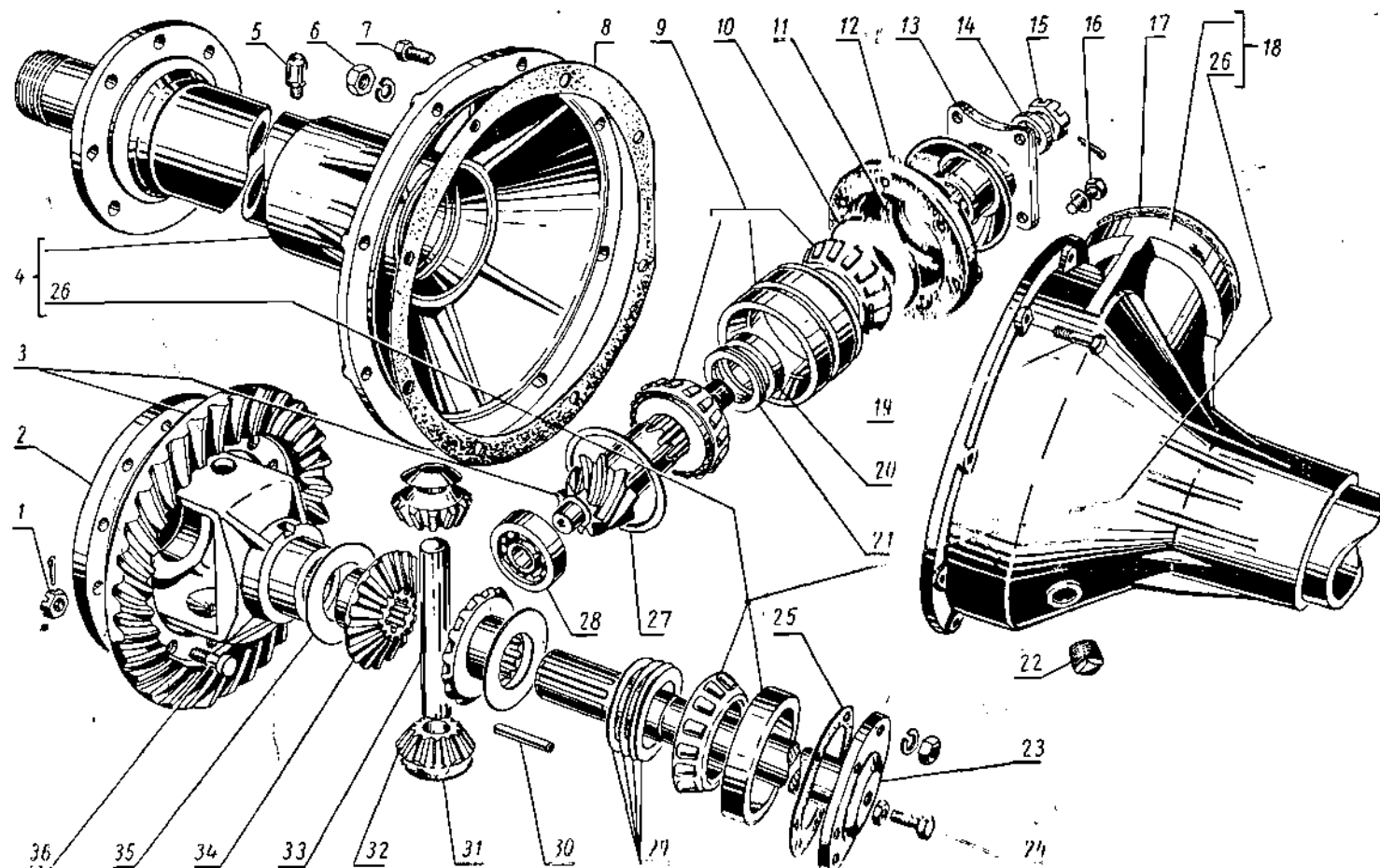
Фиг. 51. Главная передача и дифференциал переднего и заднего мостов; картер и полуоси заднего моста.
