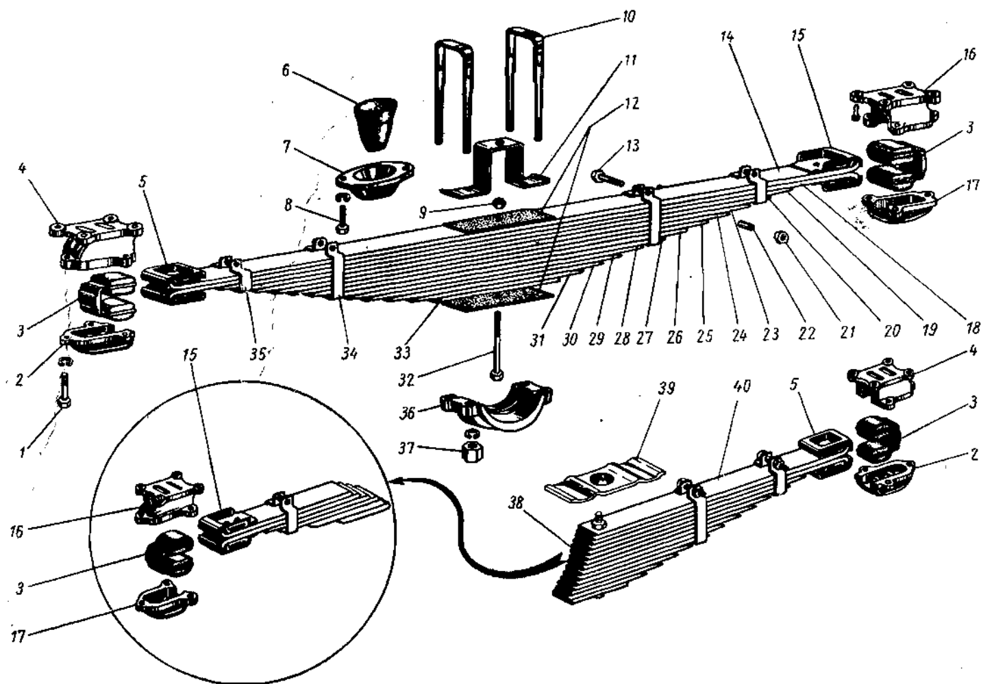
Фиг. 59. Передние и задние рессоры автомобилей УАЗ-450, УАЗ-450А и УАЗ-450Д.
