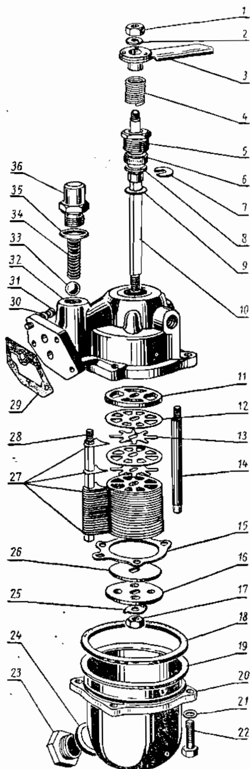
Фиг. 17. Масляный фильтр грубой очистки.
