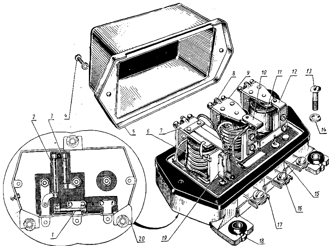
Фиг. 73. Реле-регулятор.
