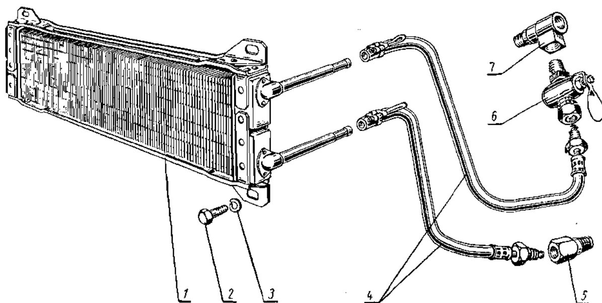
Фиг. 18. Масляный радиатор.
