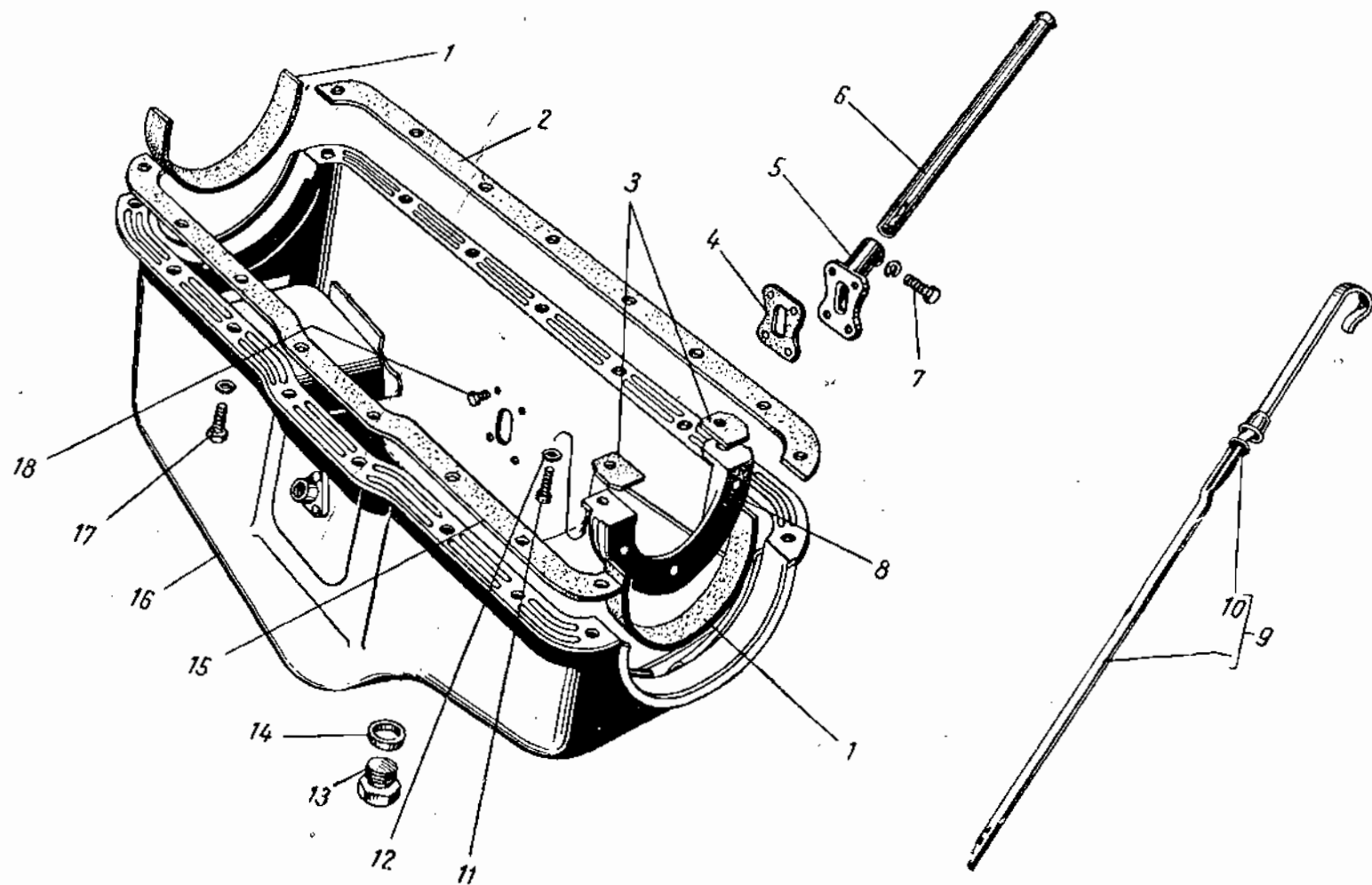
Фиг. 14. Масляный картер.
