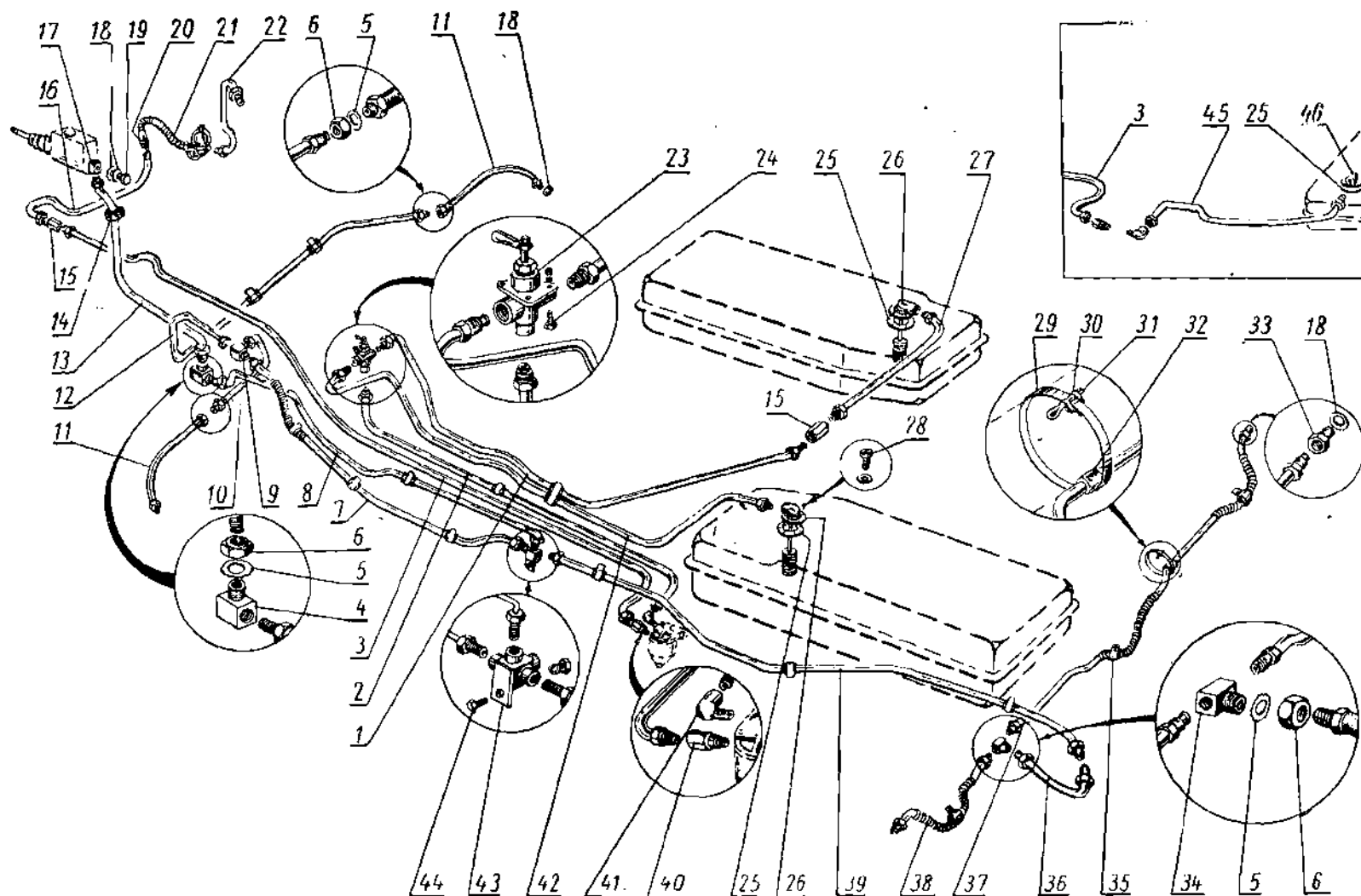
Фиг. 26. Схема системы питания и гидротормозов автомобилей УАЗ-450, УАЗ-450А и УАЗ-450Д. Примечание. Поз. 4—14, 17, 18, 19, 29—39, 43 и 44 см. в подгруппе 3506.
