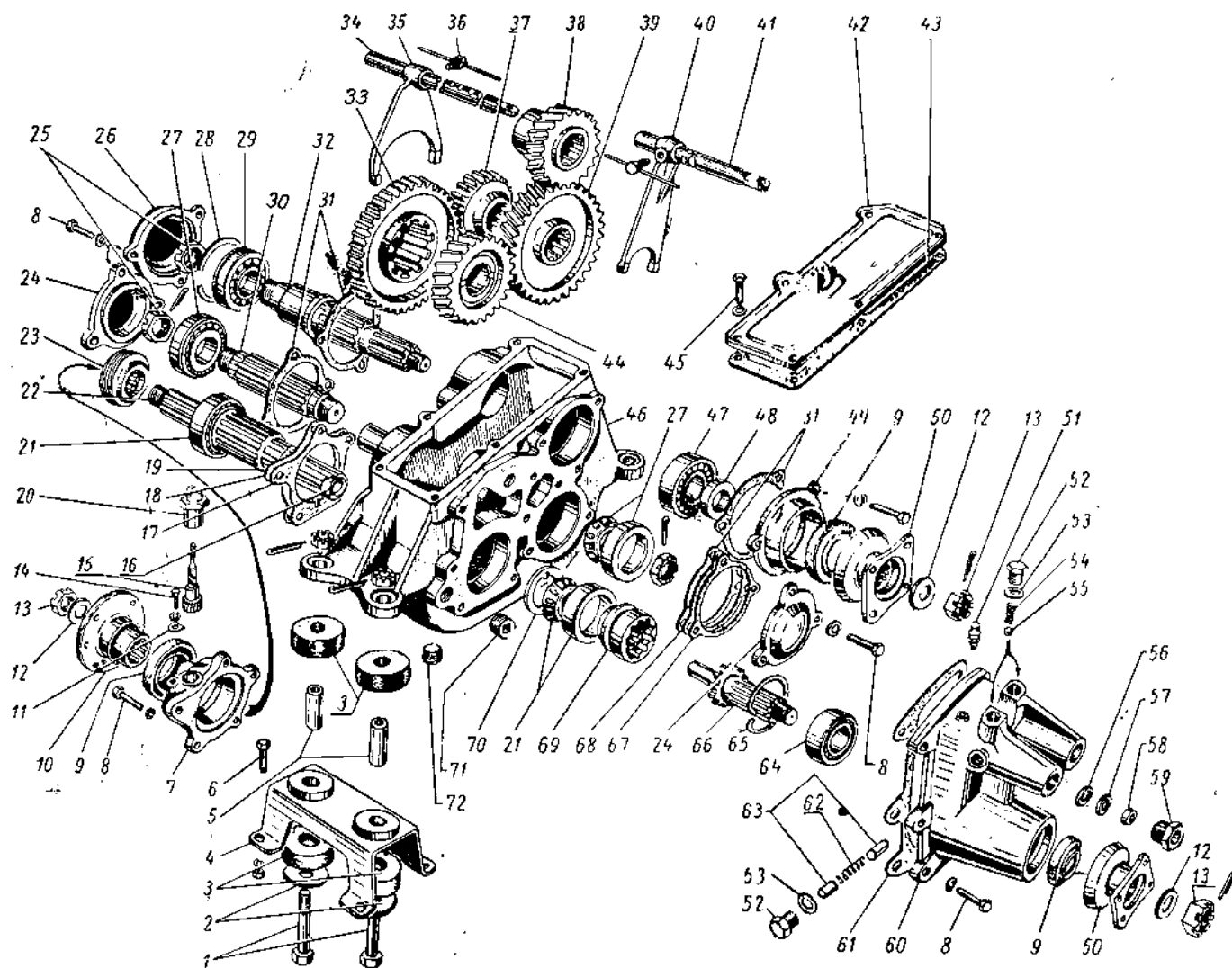
Фиг. 48. Раздаточная коробка автомобилей УАЗ-450, УАЗ-450А и УАЗ-450Д
