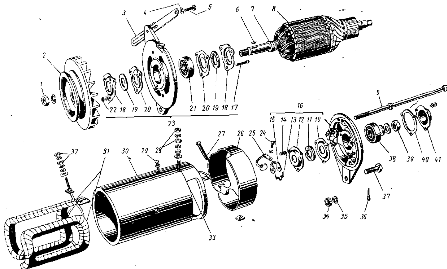
Фиг. 72. Генератор автомобилей УАЗ-450, УАЗ-450А и УАЗ-450Д.
