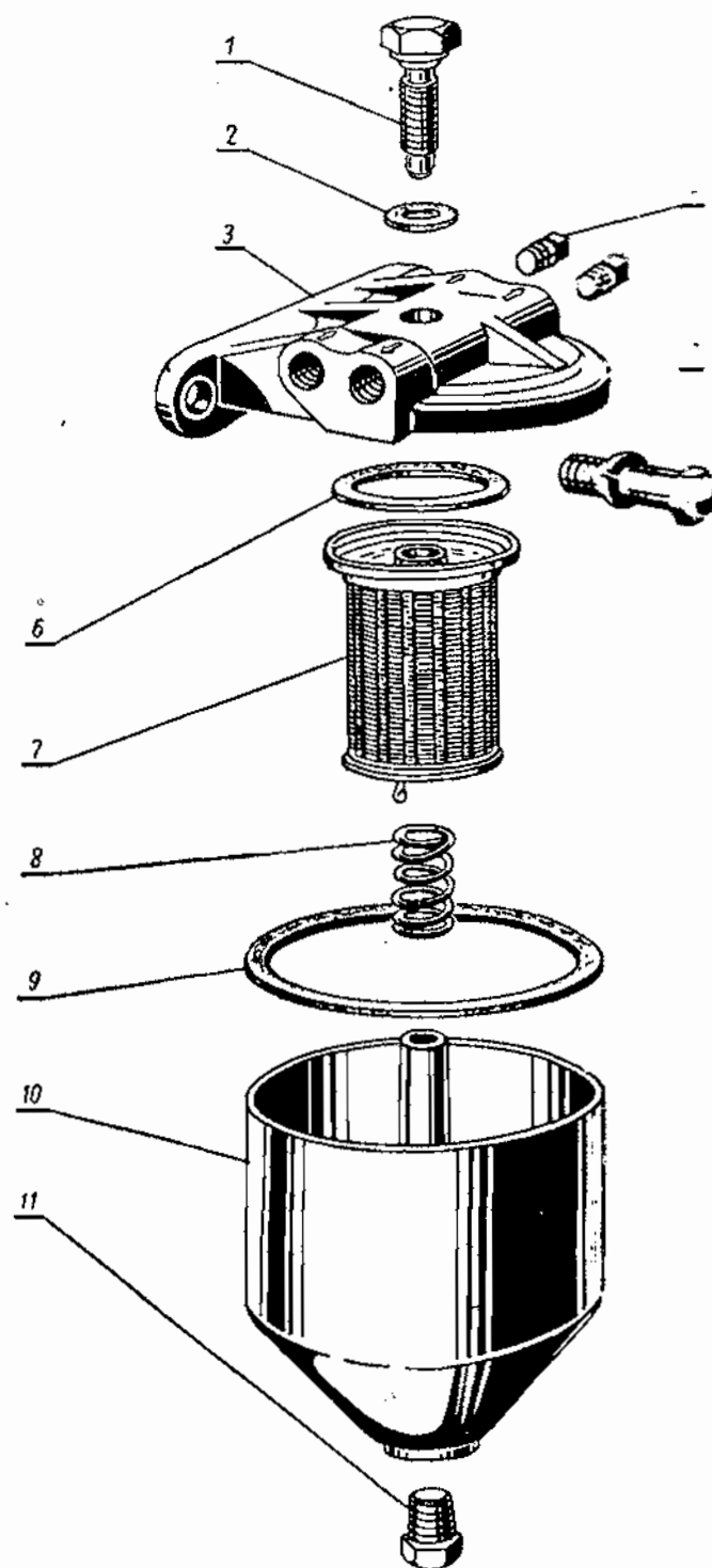
Фиг. 27. Бензиновый отстойник.
