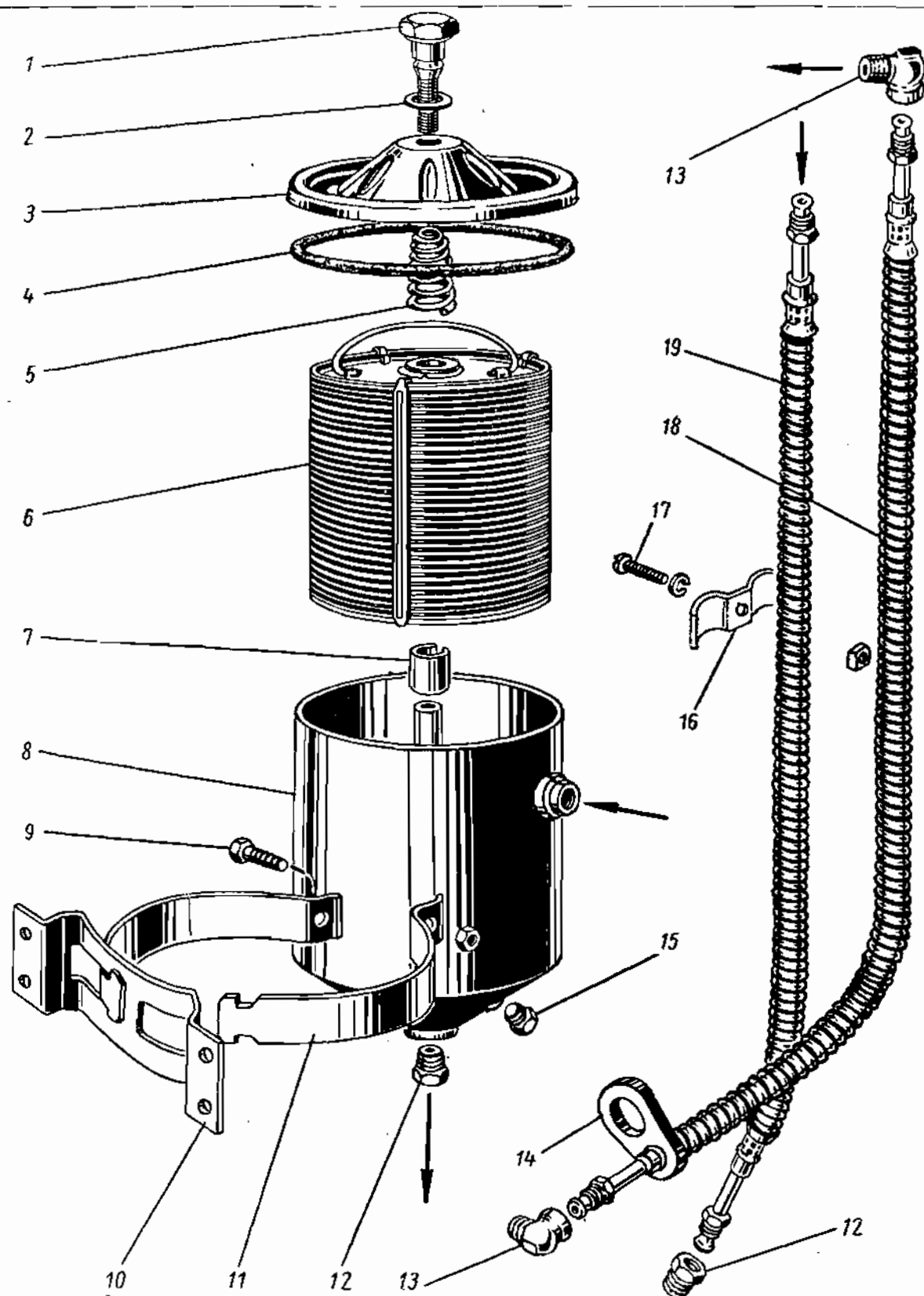
Фиг. 20. Масляный фильтр тонкой очистки.
