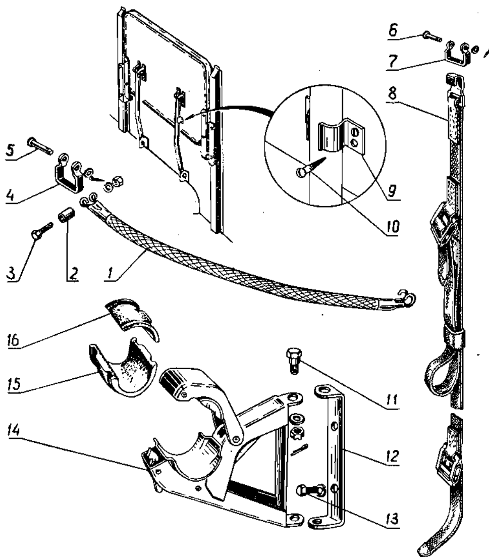
Фиг. 104. Специальное оборудование автомобиля УАЗ-450А.
