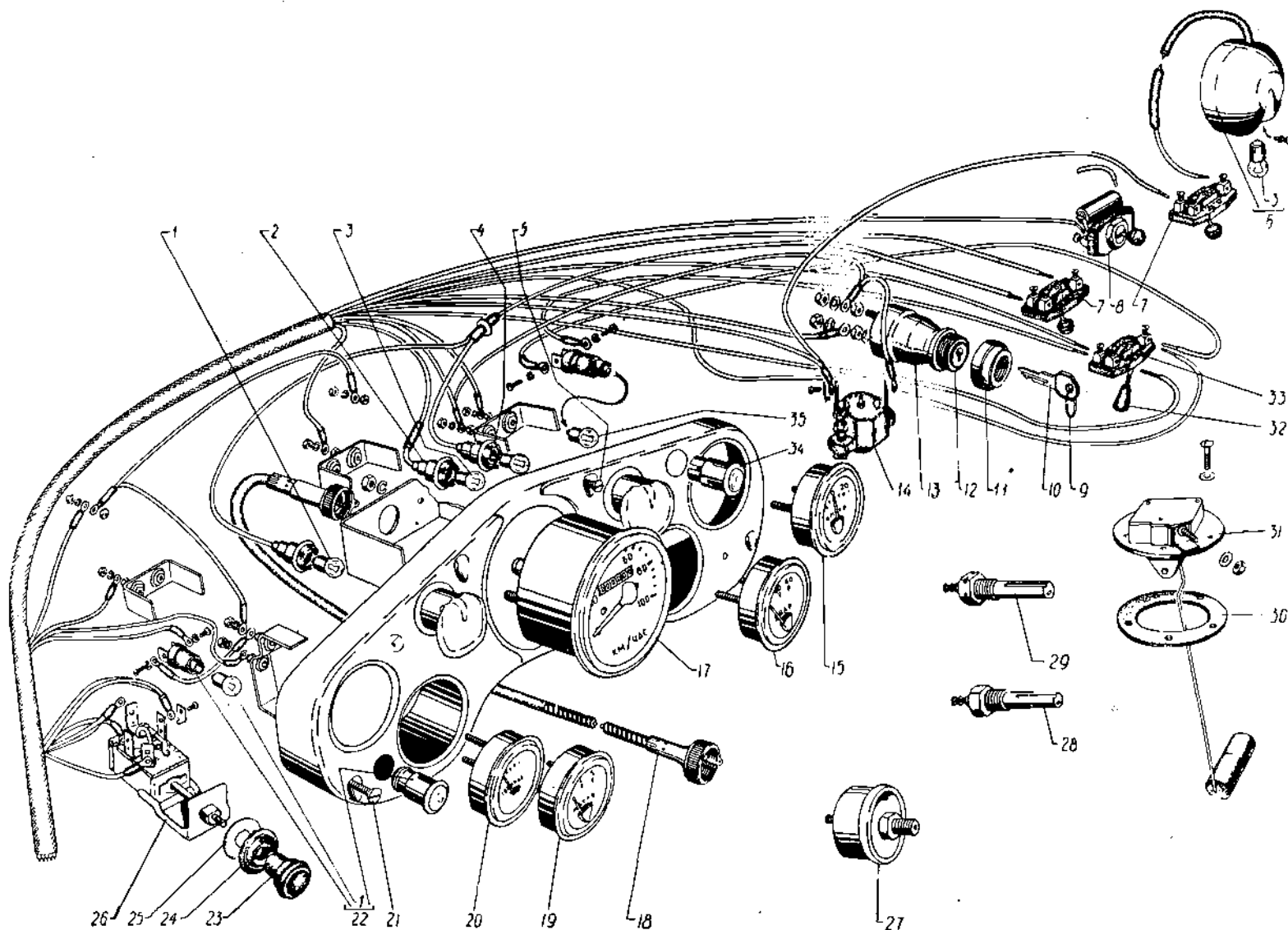
Фиг. 86. Щиток приборов и приборы автомобилей ГАЗ-69 и ГАЗ-69А
