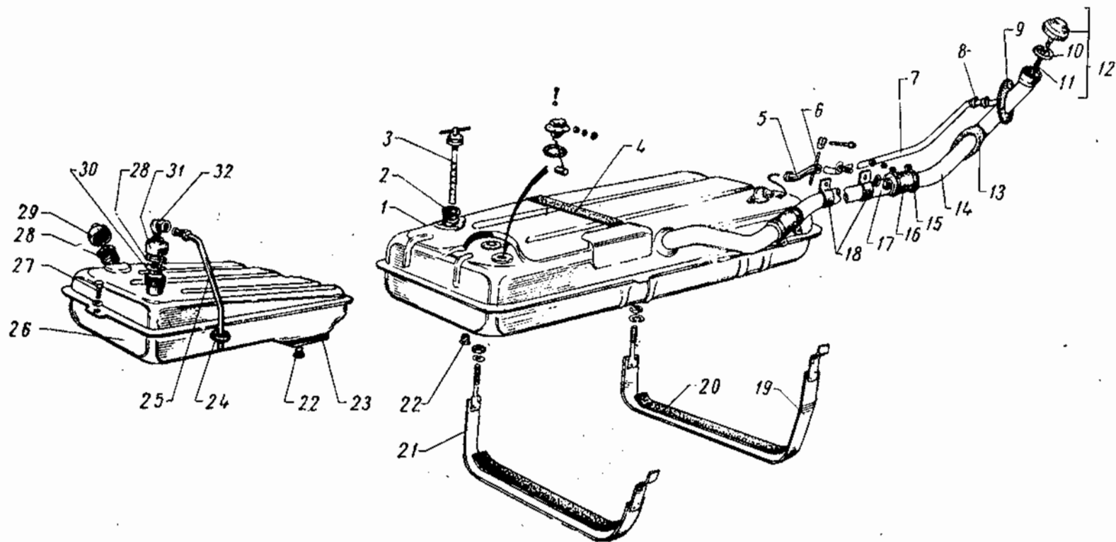
Фиг. 21. Бензиновый бак автомобиля ГАЗ-69.
