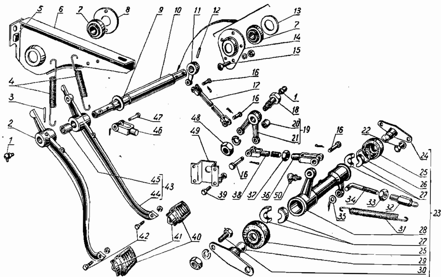
Фиг. 42. Привод выключения сцепления и тормозная педаль автомобилей УАЗ-450, УАЗ-450А и УАЗ-450Д
