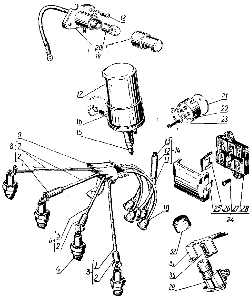
Фиг. 76. Катушка зажигания, свечи зажигания, провода, ножной переключатель света, подкапотная лампа, штепсельная розетка и блок предохранителей.
