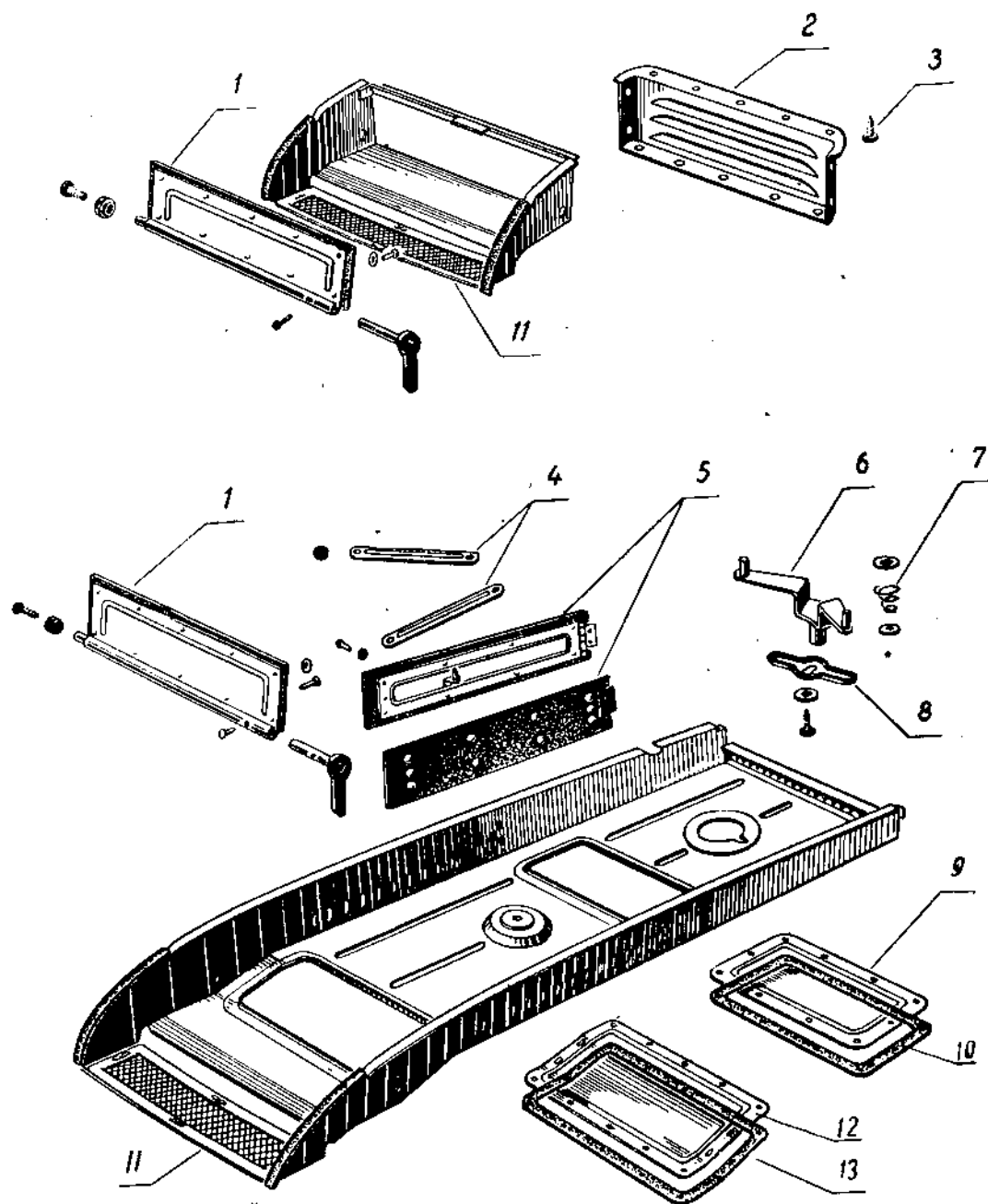
Фиг. 106. Короб вентиляции автомобилей УАЗ-450, УАЗ-450А и УАЗ-450Д.
