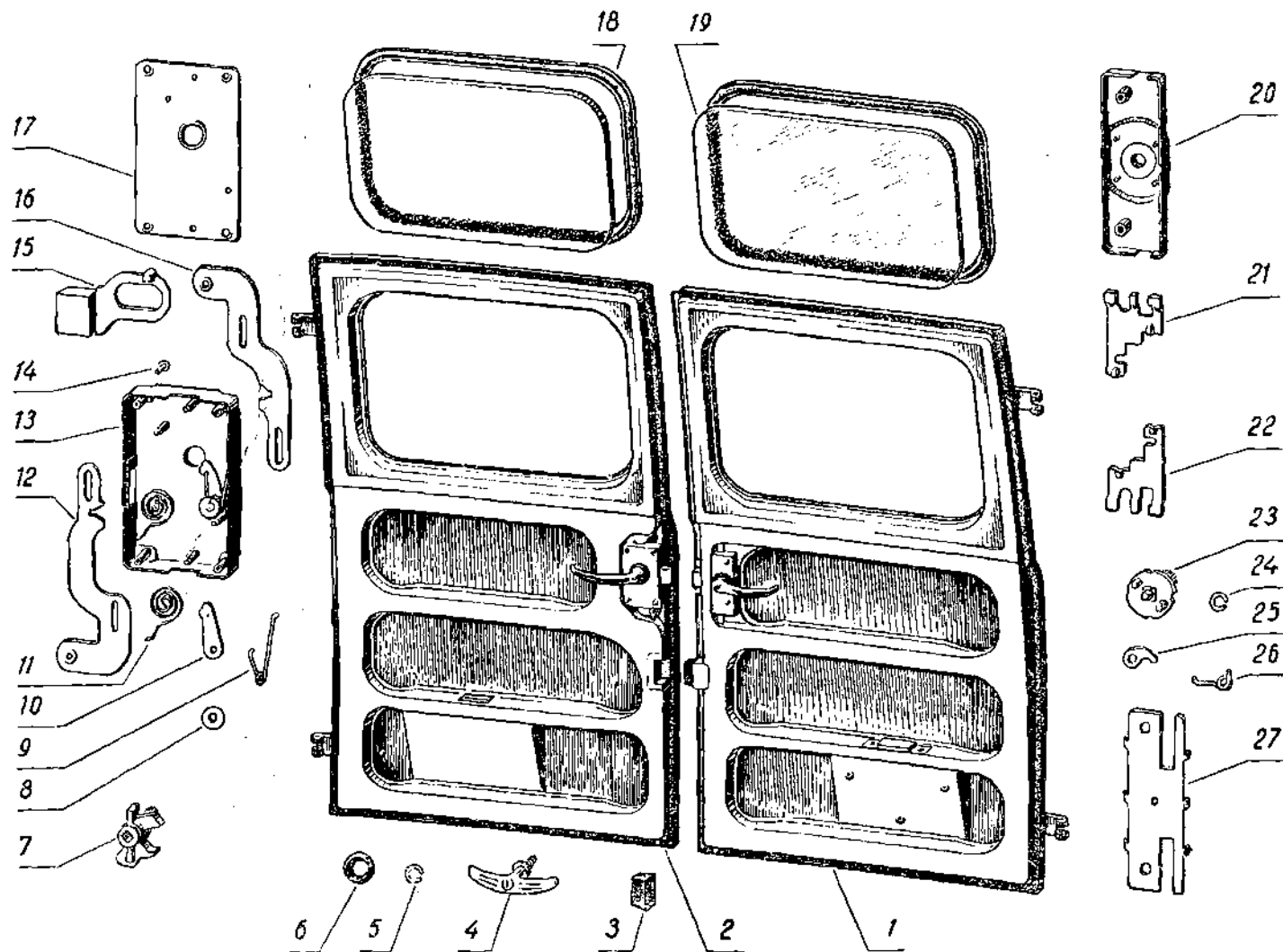
Фиг. 103. Задняя дверь с замком в сборе автомобилей УАЗ-450, УАЗ-450А и УАЗ-450Д.
