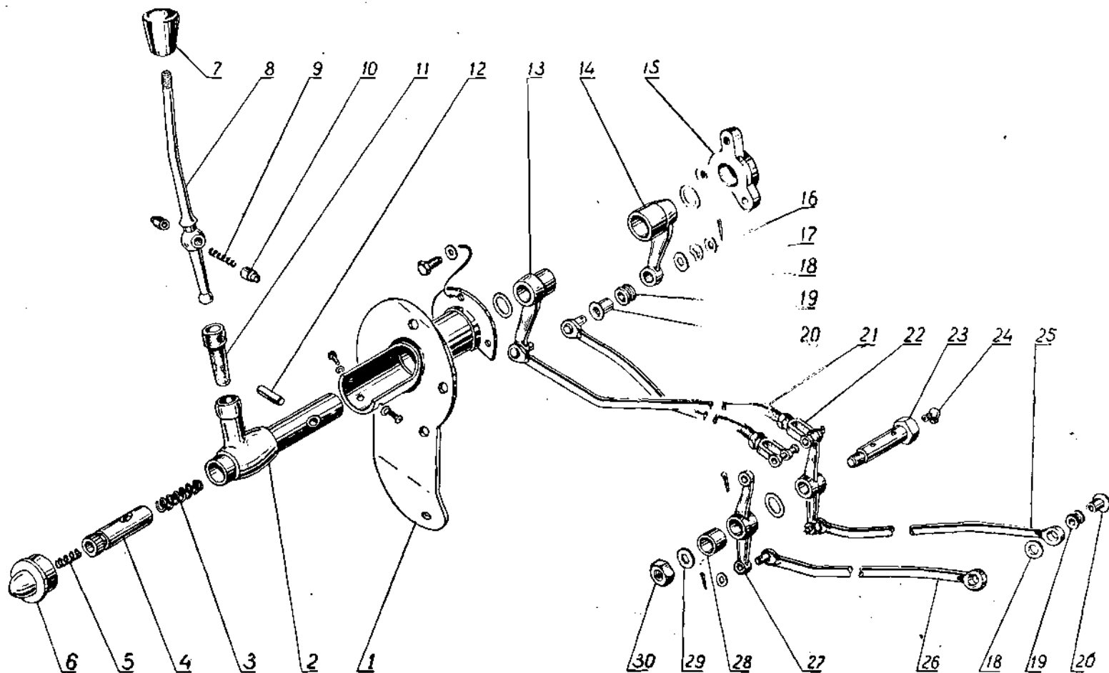
Фиг. 46. Управление коробкой передач.
