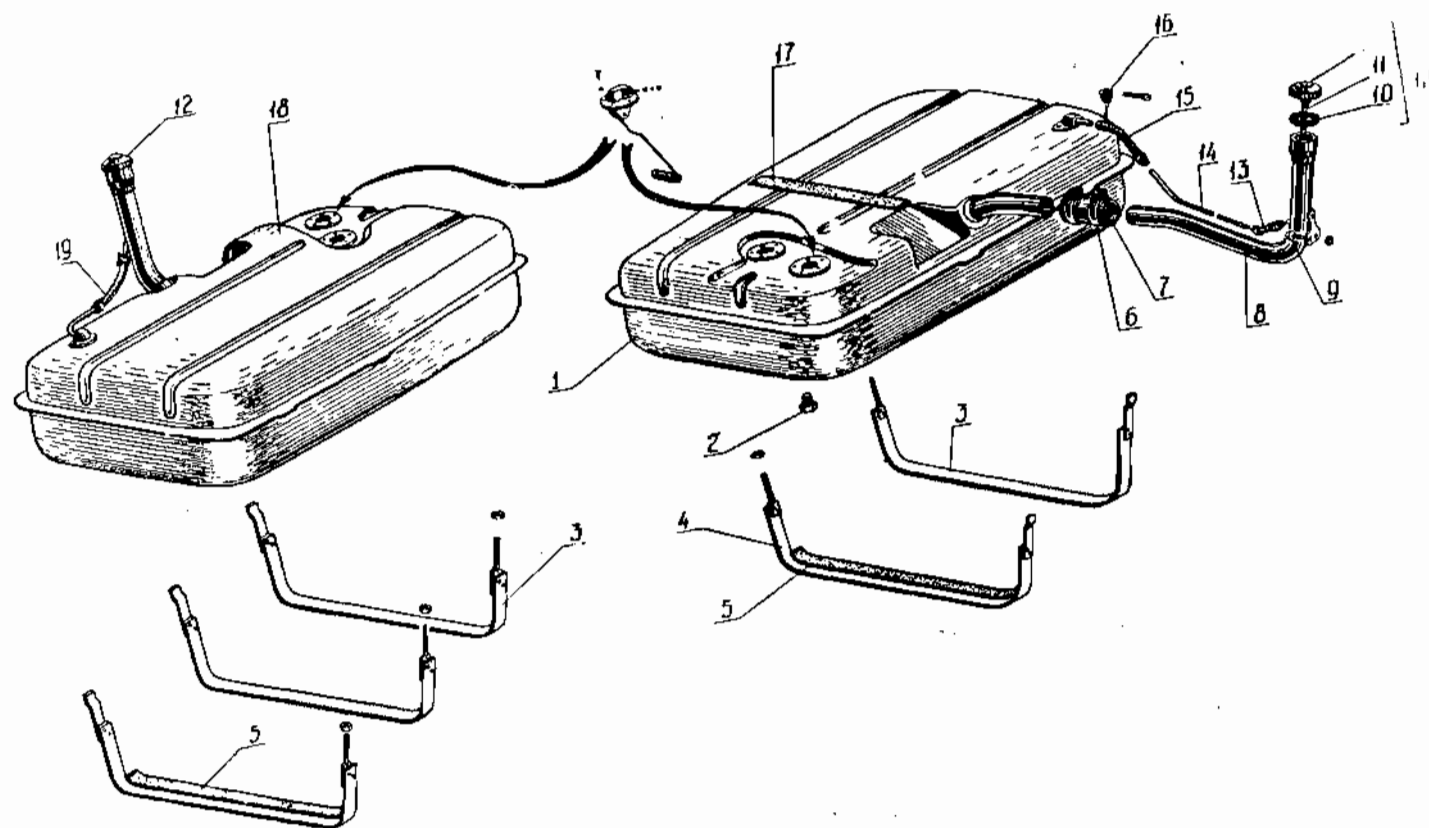
Фиг. 23. Бензиновый бак автомобилей УАЗ-450 и УАЗ-450А.
