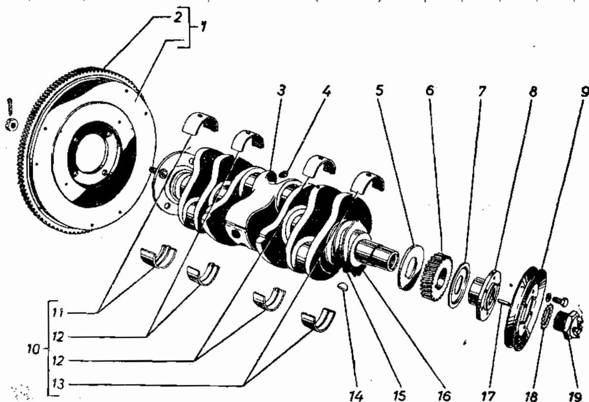
Фиг. 10. Коленчатый вал и маховик. Примечание. Поз. 10 см. в подгруппе 1000.
