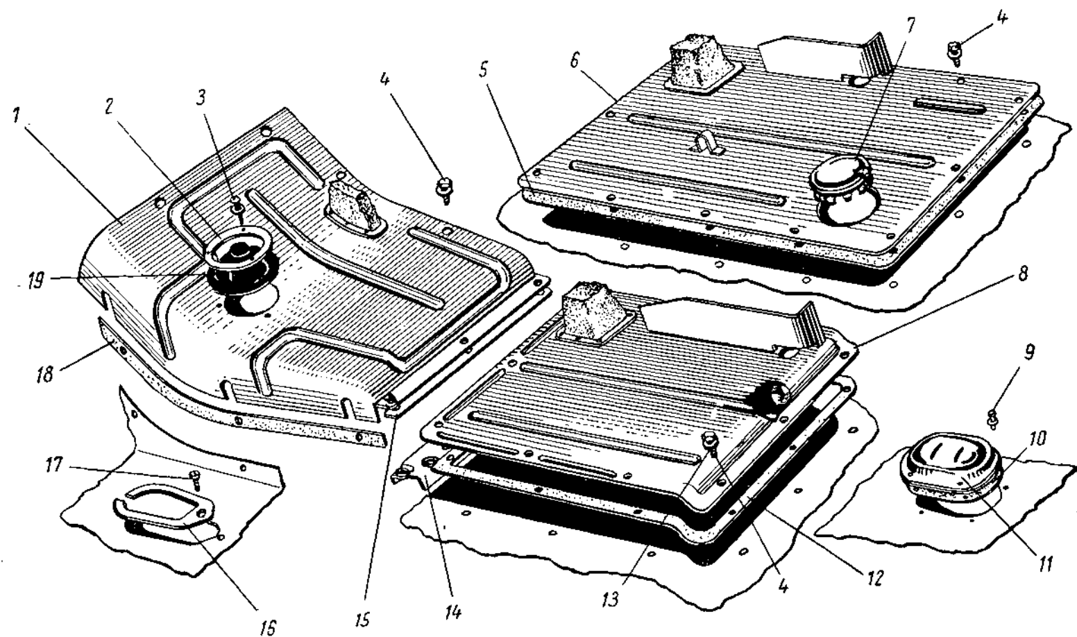
Фиг. 91. Детали пола и кожух автомобилей ГАЗ-69 и ГАЗ-69А.
