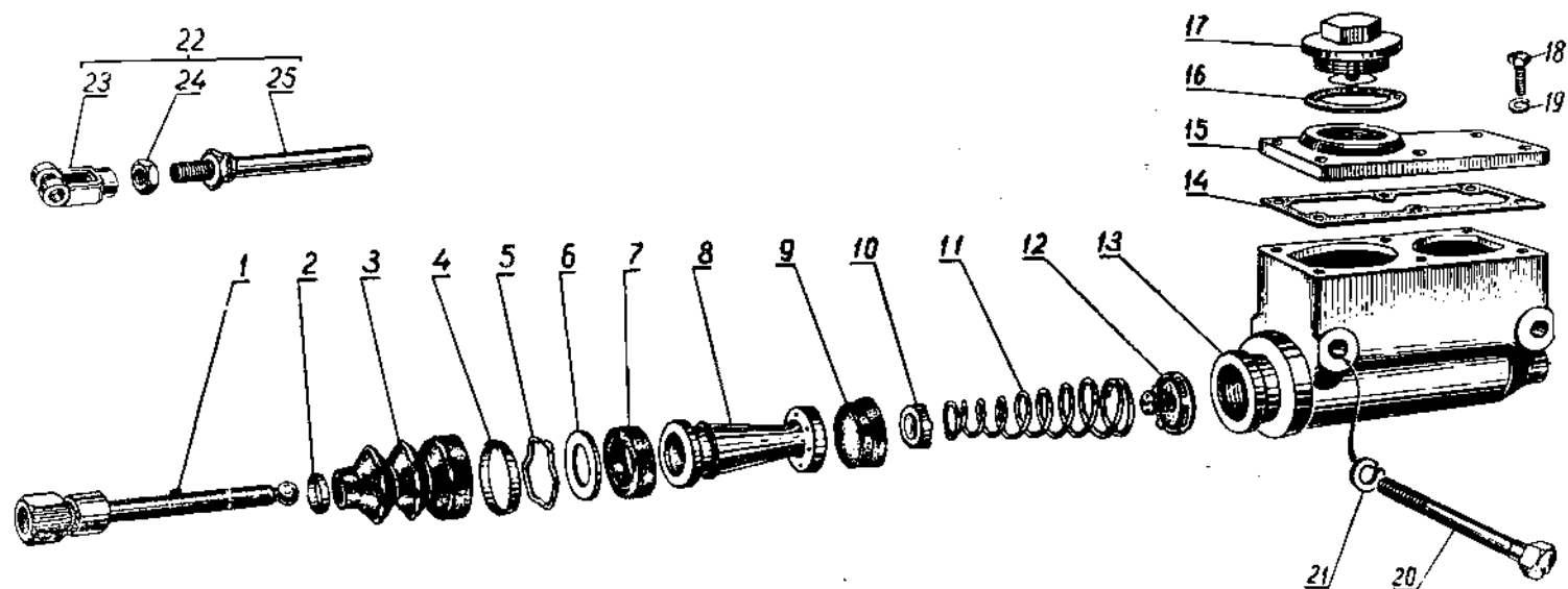
Фиг. 68. Главный цилиндр тормоза.
