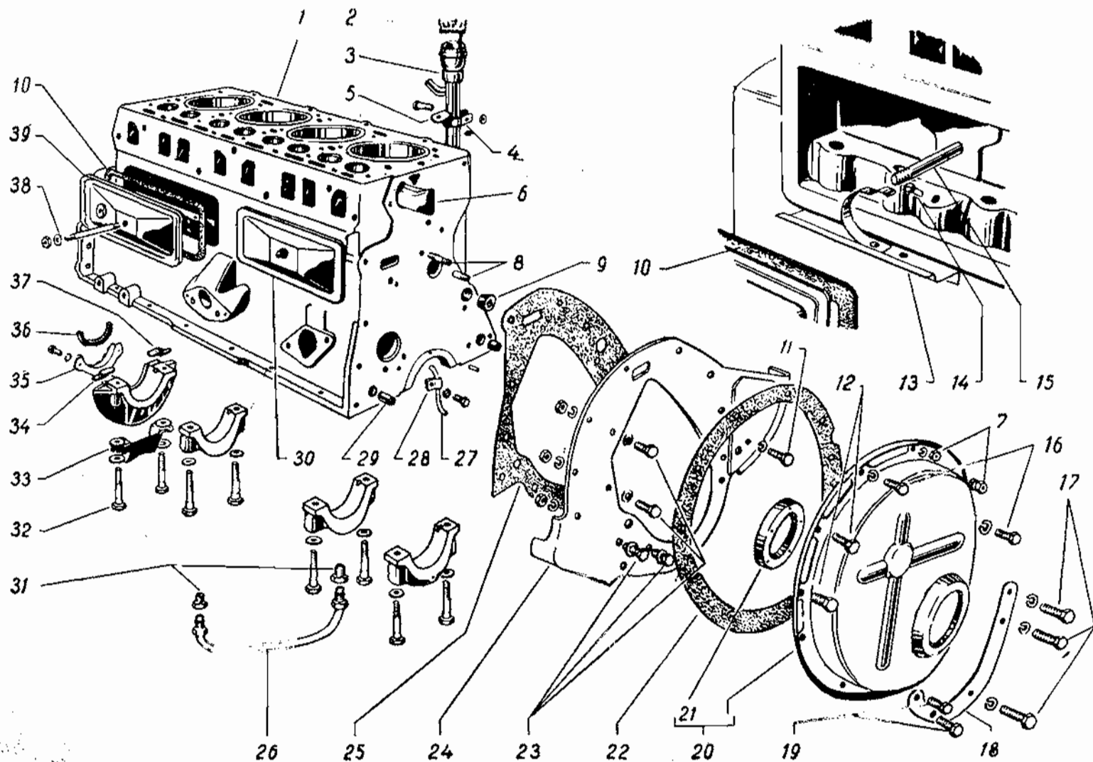
Фиг. 7. Блок цилиндров.
