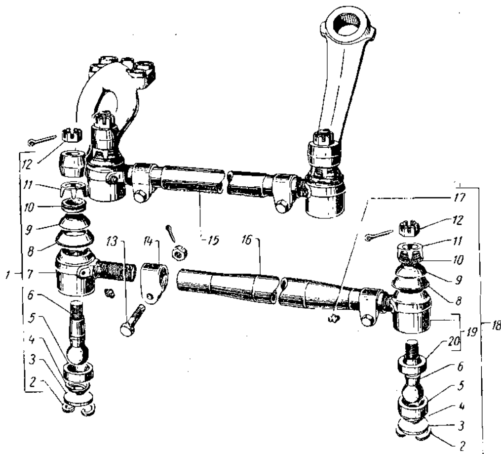
Фиг. 62. Рулевые тяги.
