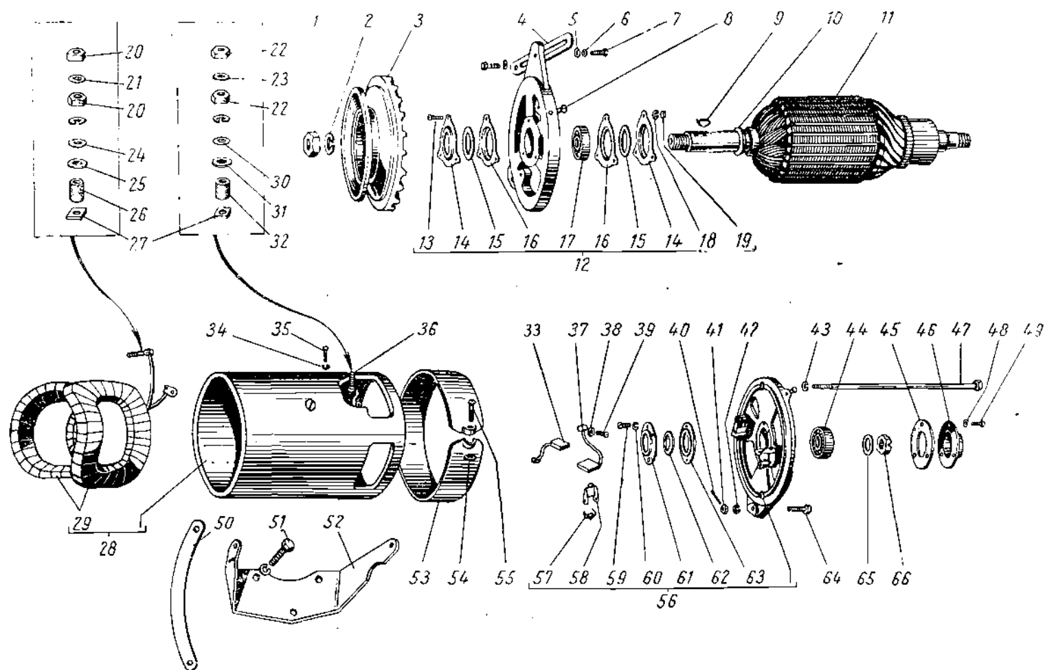
Фиг. 71. Генератор автомобилей ГАЗ-69 и ГАЗ-69А.
