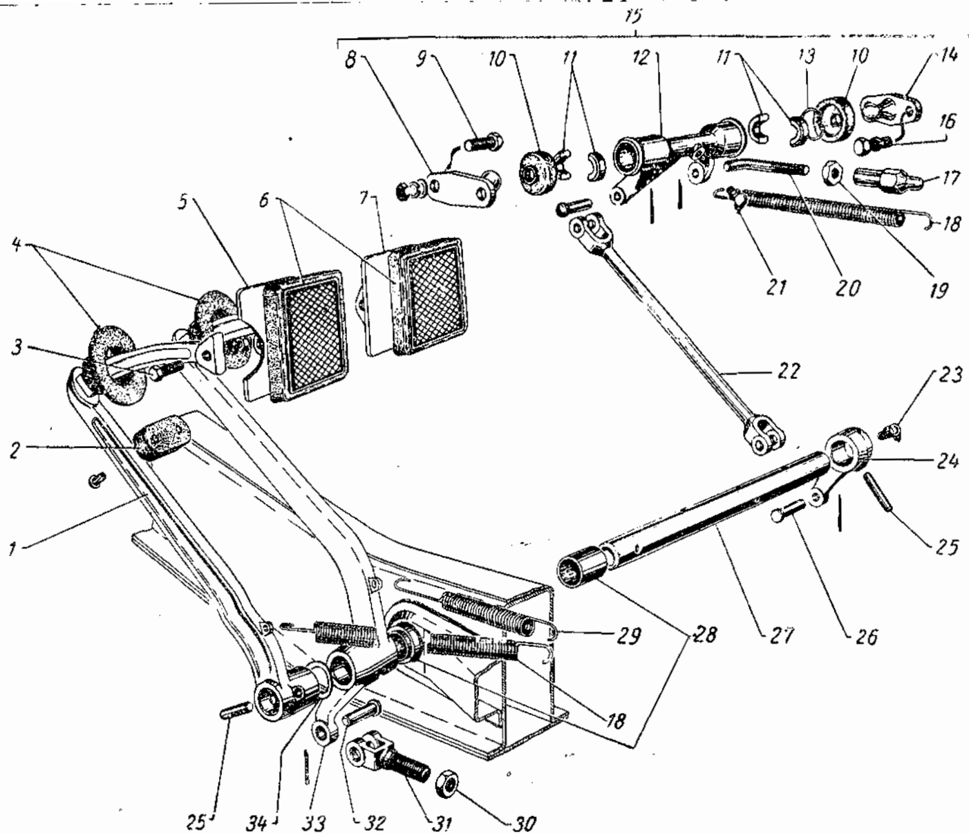
Фиг. 41. Привод выключения сцепления и тормозная педаль автомобилей ГАЗ-69 и ГАЗ-69А Примечание. Поз. 2, 3, 4, 6, 7 и 29—33 см. в подгруппе 3504.
