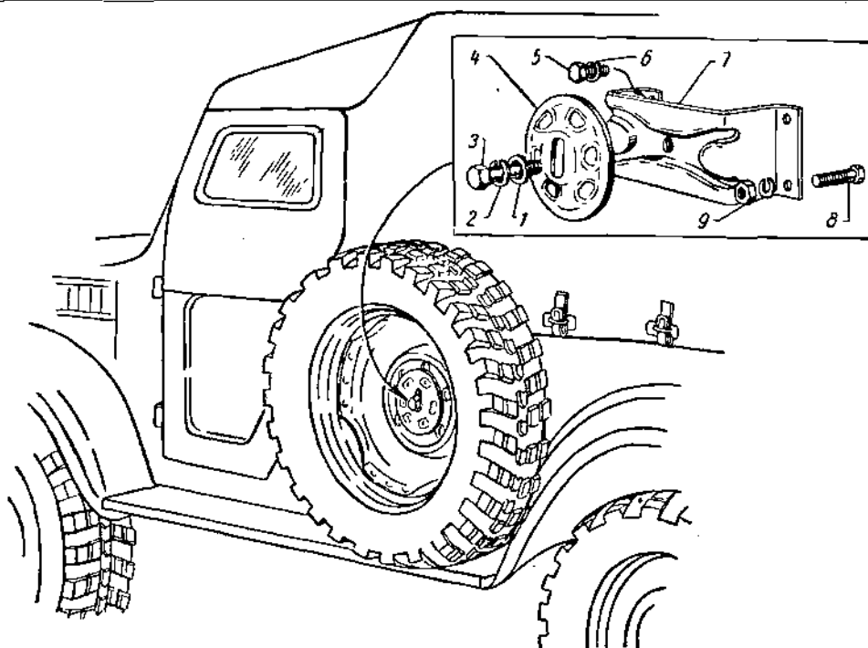
Фиг. 63. Держатель запасного колеса автомобиля ГАЗ-69.
