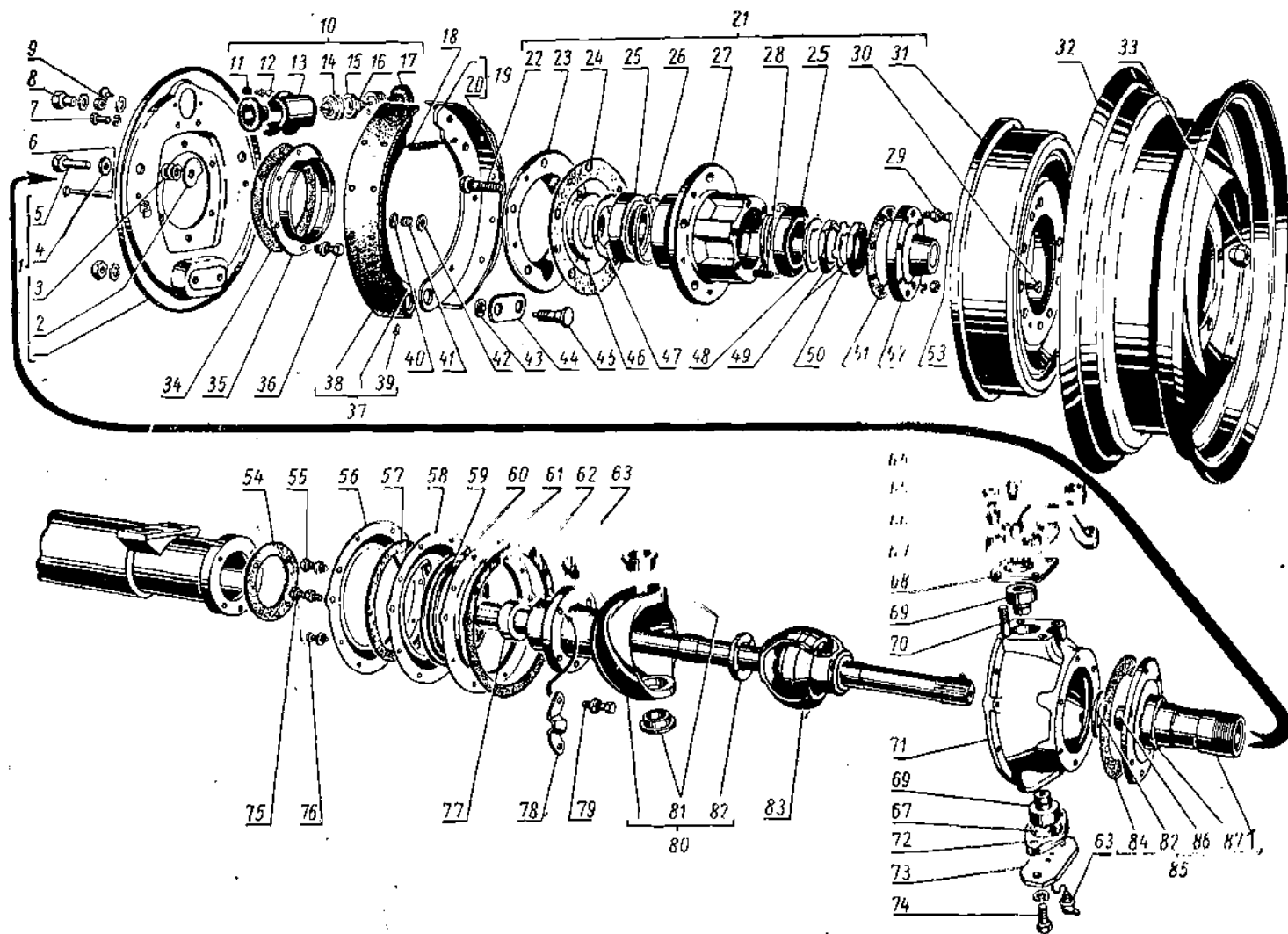
Фиг. 52. Поворотные кулаки переднего моста; колеса и ступицы; ножные тормоза.
