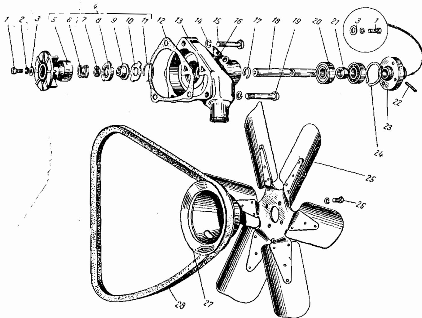
Фиг. 39. Водяной насос.
