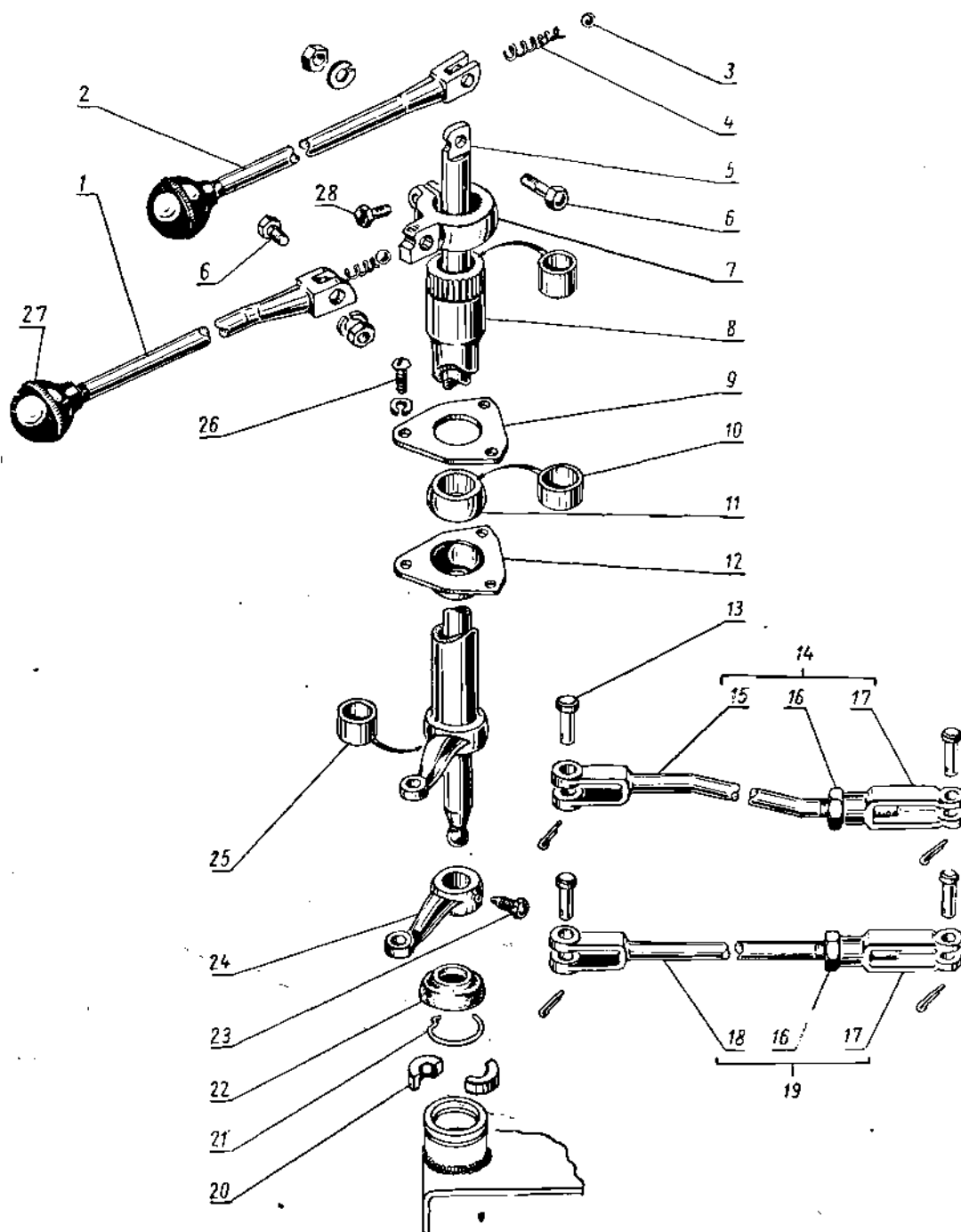
Фиг. 49. Управление раздаточной коробкой автомобилей УАЗ-450, УАЗ-450А и УАЗ-450Д.
