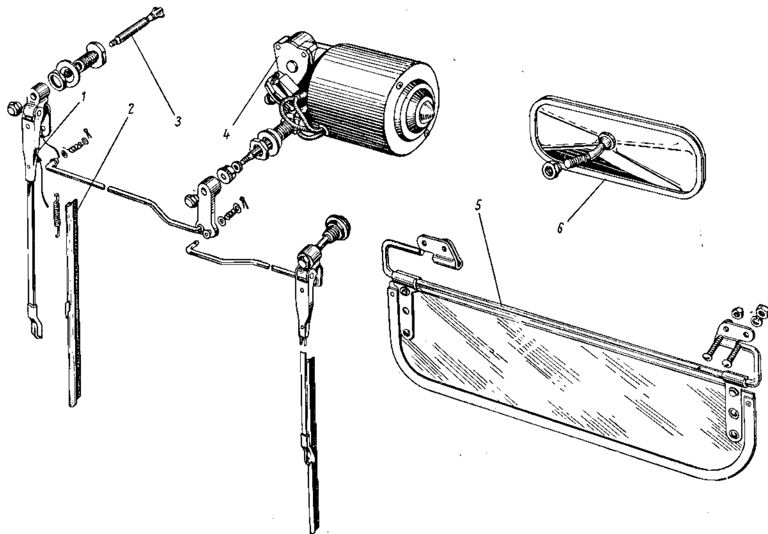
Фиг. 93. Стеклоочиститель, зеркало заднего вида и противосолнечный козырек автомобилей ГАЗ-69 и ГАЗ-69А. Примечание. 1) поз. 6 см. в подгруппе 8201; 2) поз. 5 см. в подгруппе 8204.
