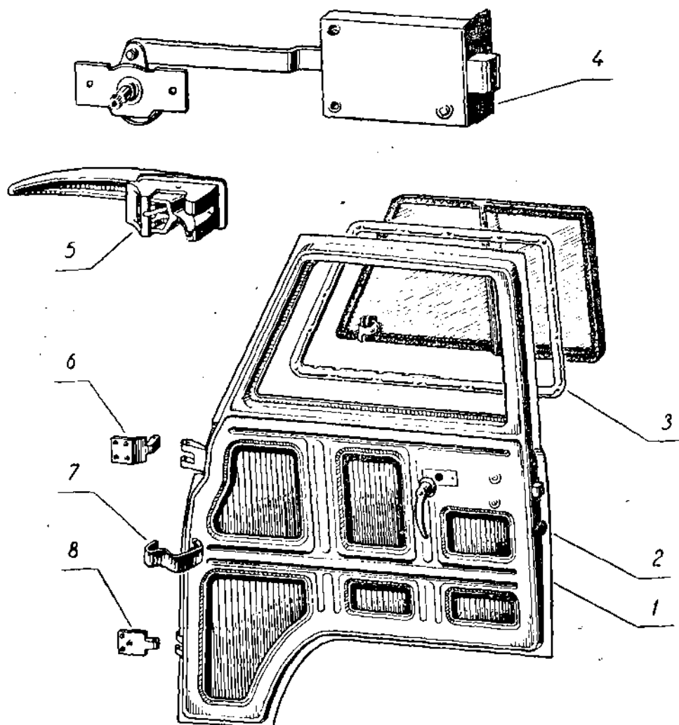
Фиг. 102 Передняя дверь автомобилей УАЗ-450, УАЗ-450А и УАЗ-450Д.
