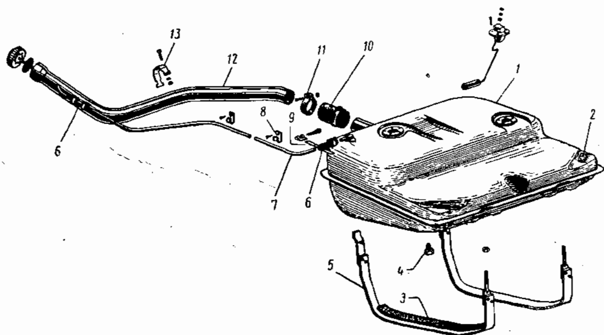
Фиг. 24. Бензиновый бак автомобиля УАЗ-450Д.
