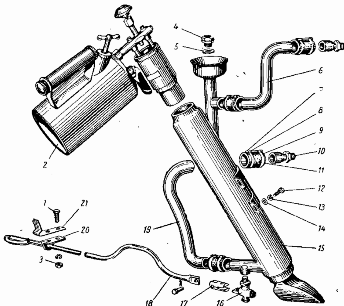
Фиг. 19. Пусковое оборудование двигателя автомобилей ГАЗ-69 и ГАЗ-69А.
