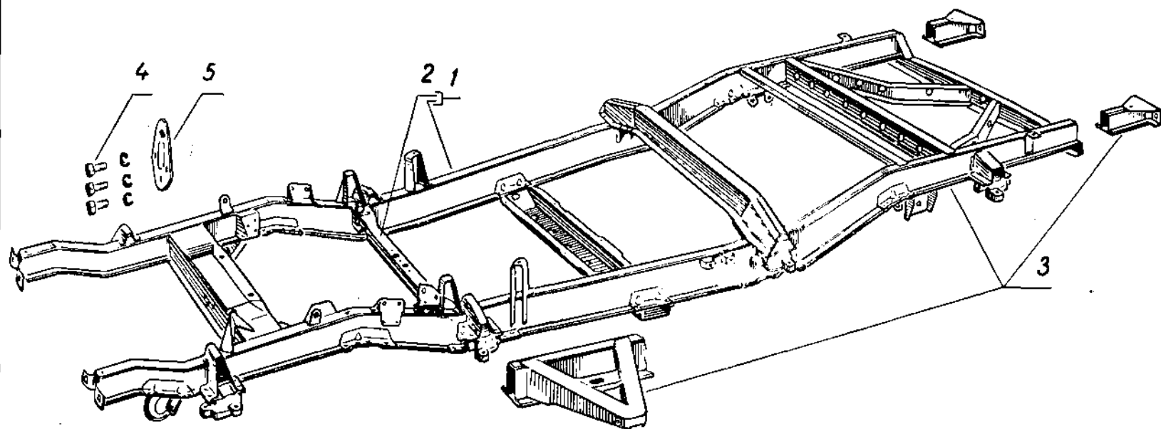
Фиг. 54. Рама автомобилей УАЗ-450, УАЗ-450А и УАЗ-450Д.
