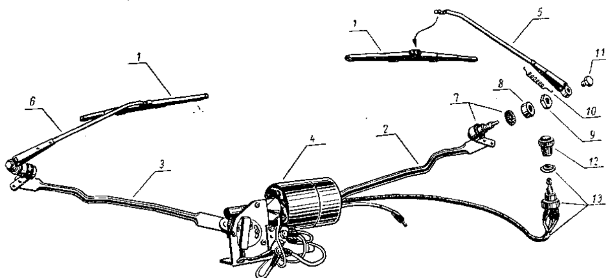
Фиг. 94. Стеклоочиститель автомобилей УАЗ-450, УАЗ-450А и УАЗ-450Д.
