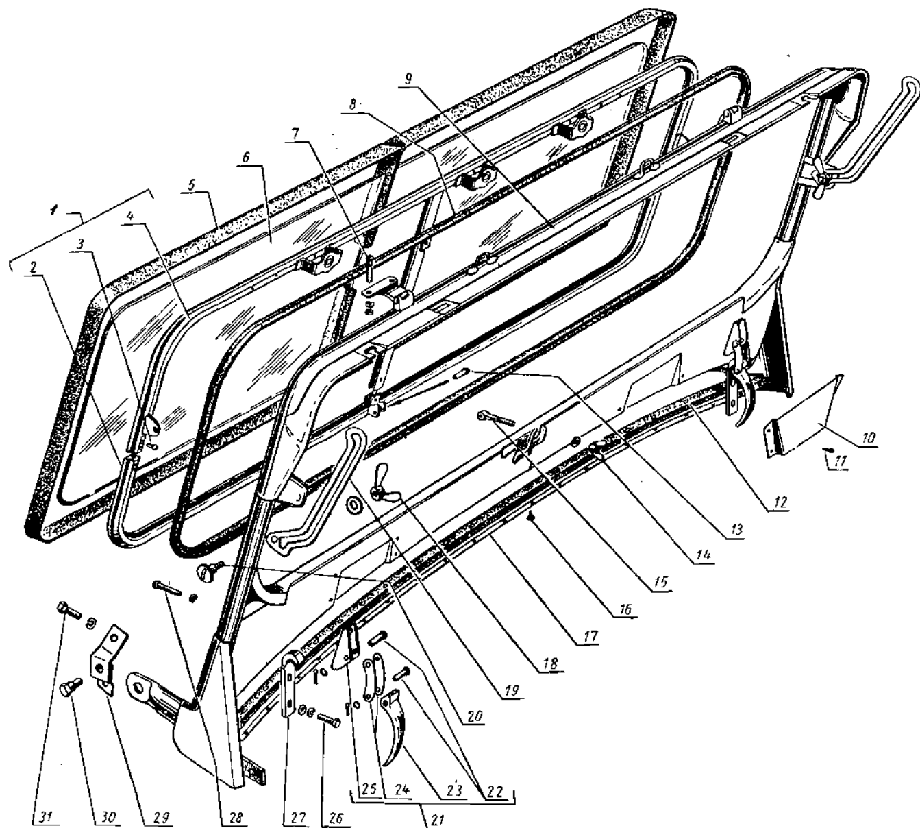
Фиг. 92. Ветровое окно автомобилей ГАЗ-69 и ГАЗ-69А. Примечание. Поз. 10 и 11 см. в подгруппе 8102.
