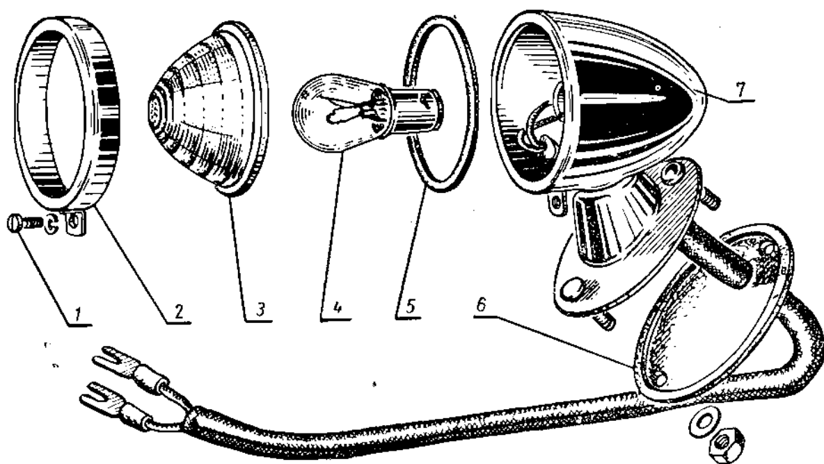
Фиг. 80. Подфарник автомобилей ГАЗ-69 и ГАЗ-69А.
