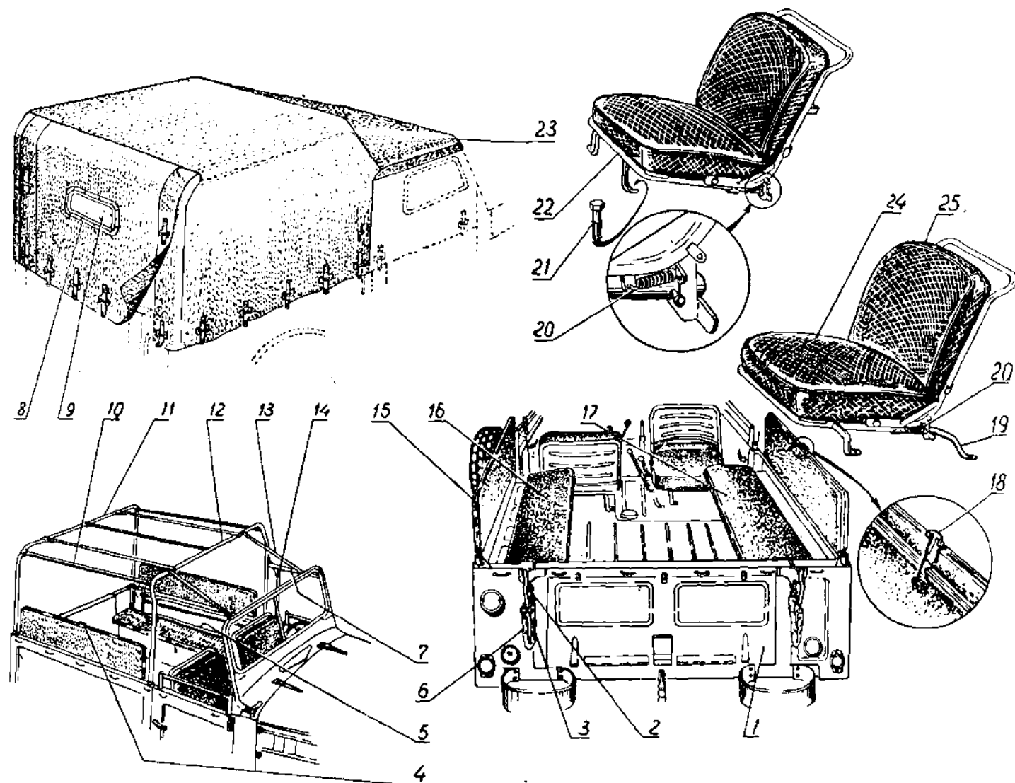
Фиг. 98. Детали кузова автомобиля ГАЗ-69.
