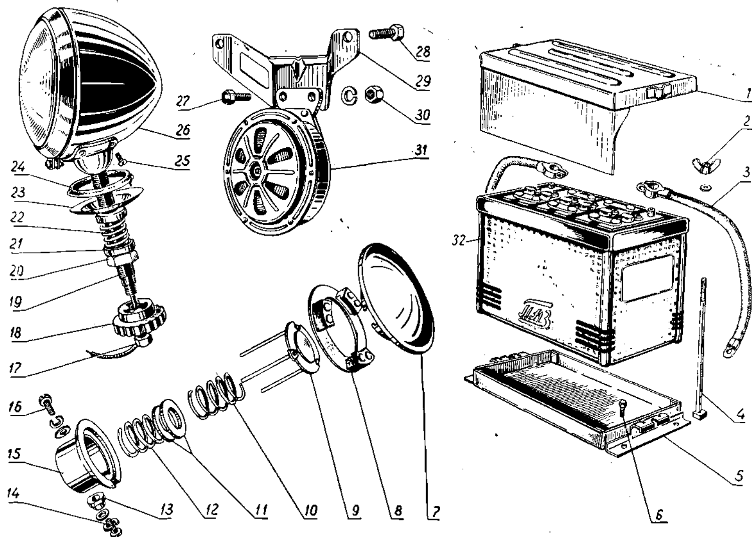
Фиг. 75. Аккумуляторная батарея; поворотная фара, сигнал и кнопка сигнала автомобилей УАЗ-450, УАЗ-450А и УАЗ-450Д.
