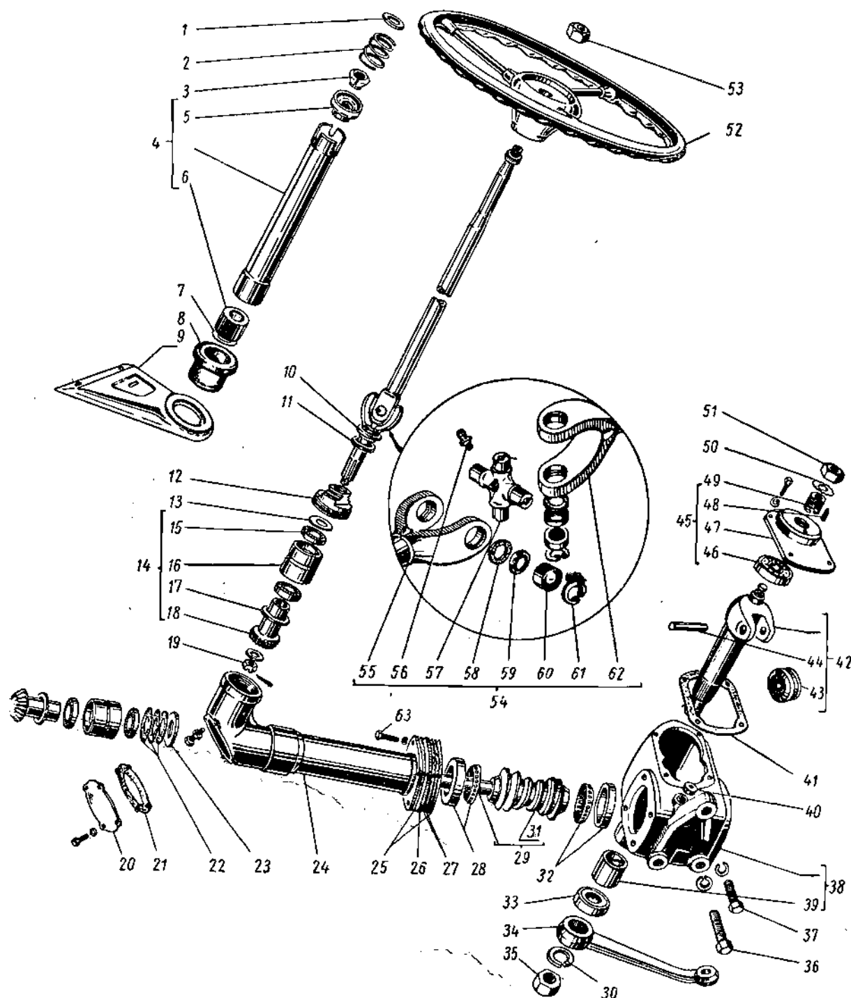
Фиг. 67. Рулевое управление автомобилей УАЗ-450, УАЗ-450А и УАЗ-450Д.
