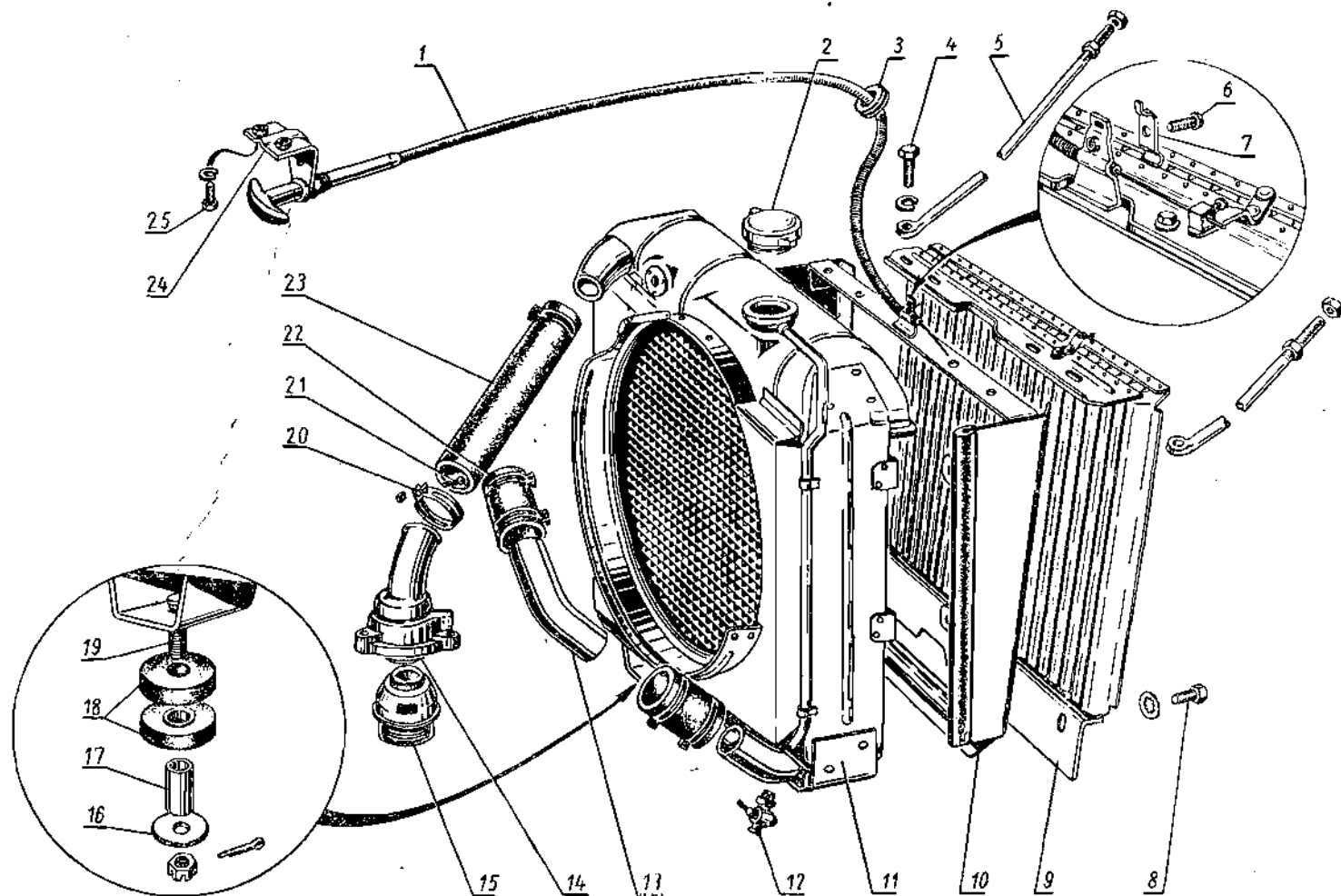
Фиг. 38. Радиатор автомобилей УАЗ-450, УАЗ-450А и УАЗ-450Д.
