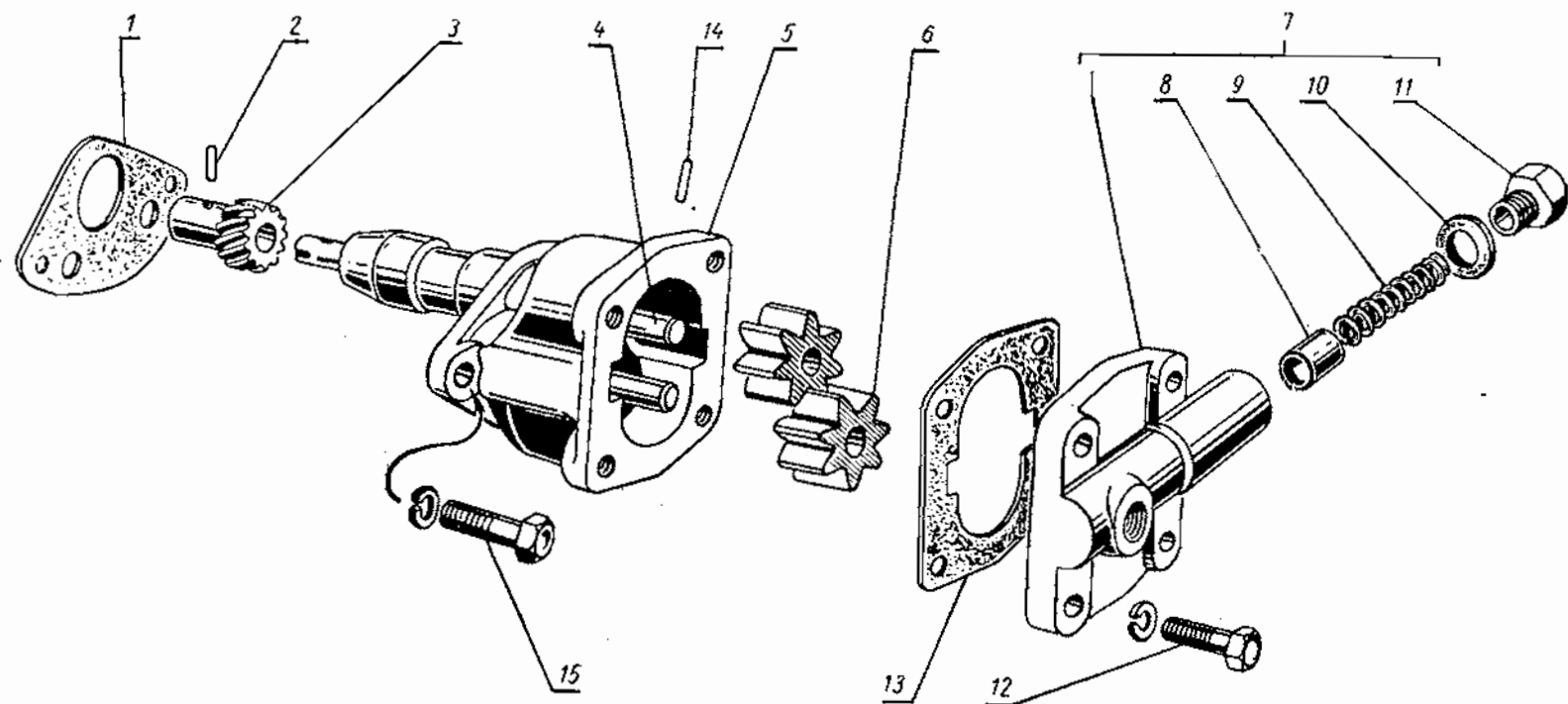
Фиг. 16. Масляный насос.
