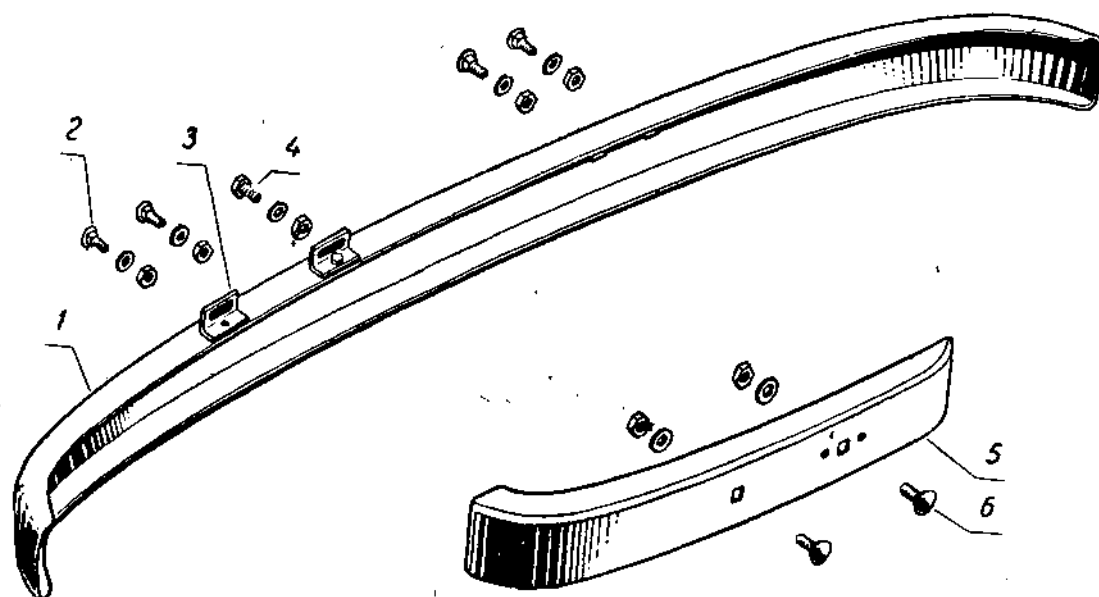
Фиг. 56. Буферы автомобилей УАЗ-450, УАЗ-450А и УАЗ-450Д.
