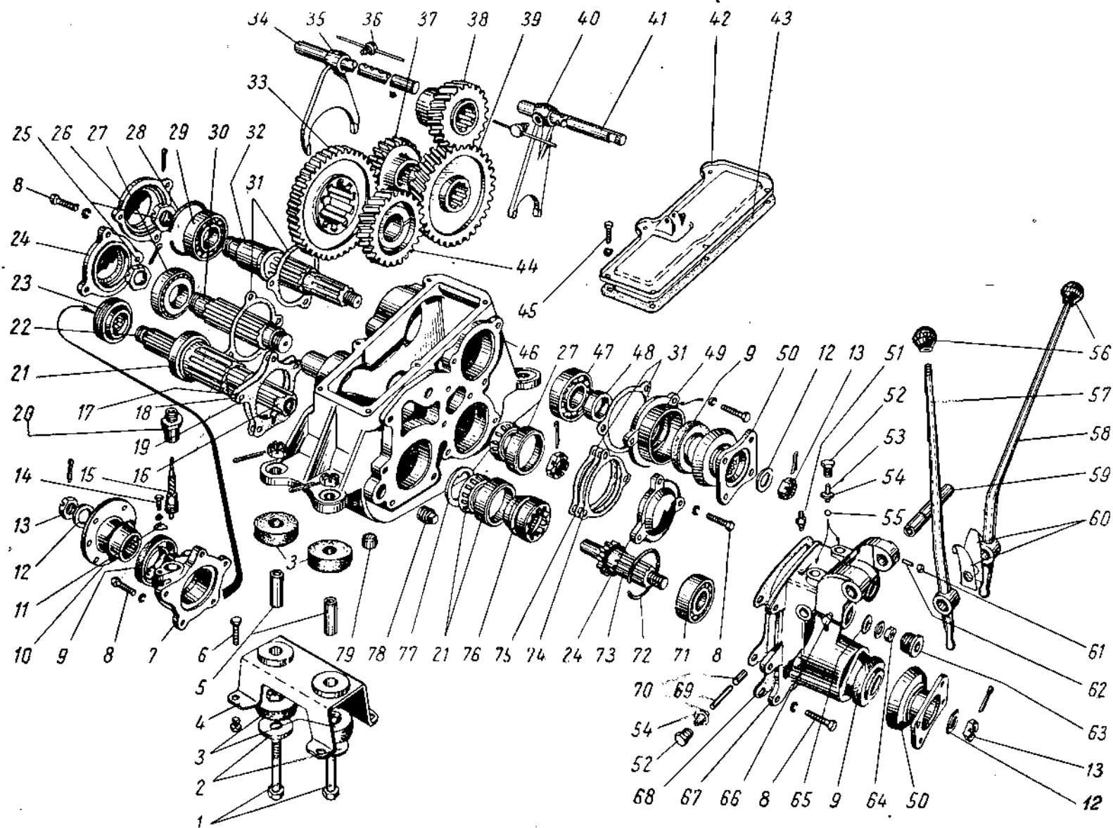
Фиг. 47. Раздаточная коробка автомобилей ГАЗ-69 и ГАЗ-69А.
