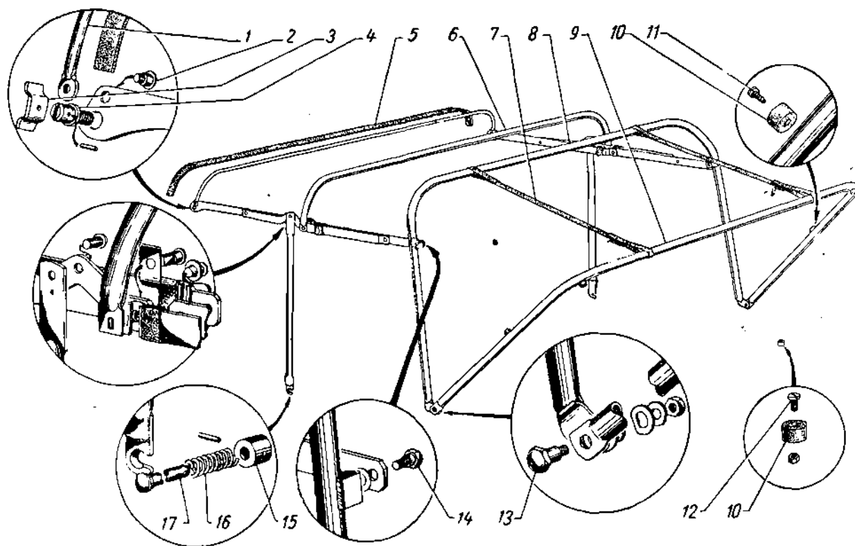
Фиг. 99. Крепление тента автомобиля ГАЗ-69А.
