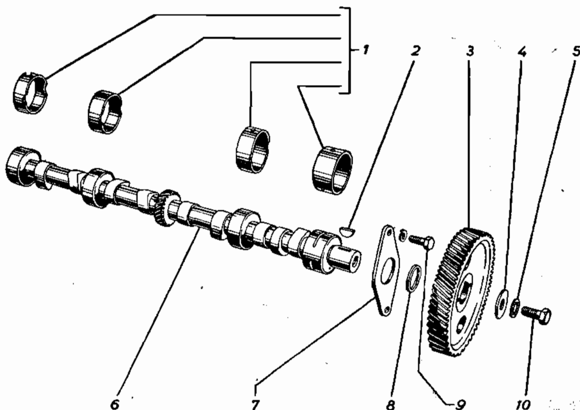
Фиг. 11. Распределительный вал.
