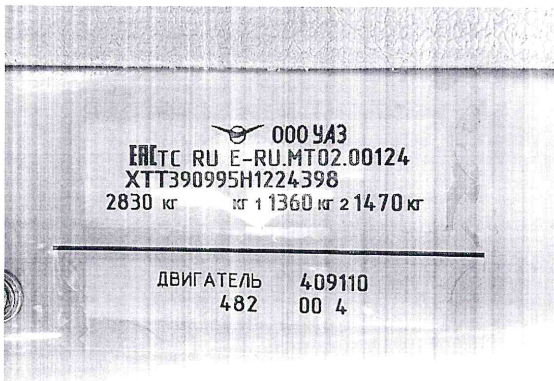
Рис. А.1 Табличка изготовителя, код VIN транспортного средства.
