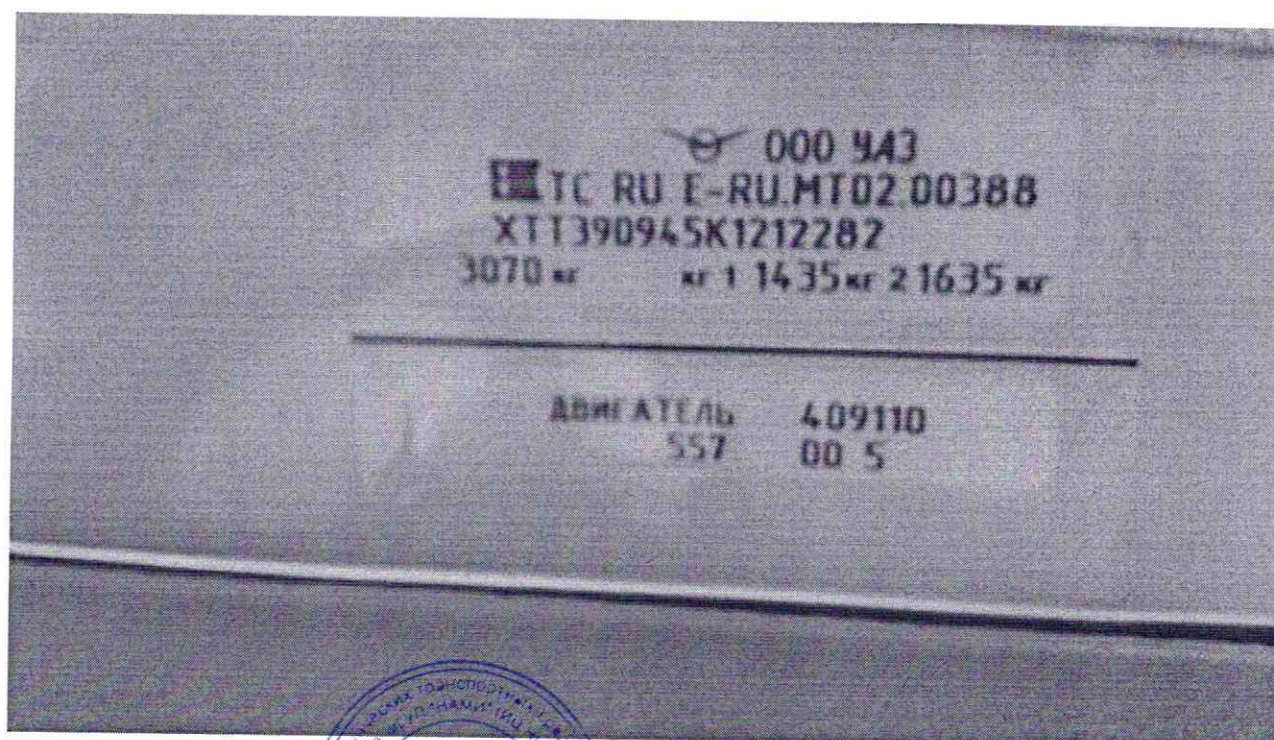
Табличка изготовителя с кодом VIN транспортного средства УАЗ, тип 3909, модификация 390945
